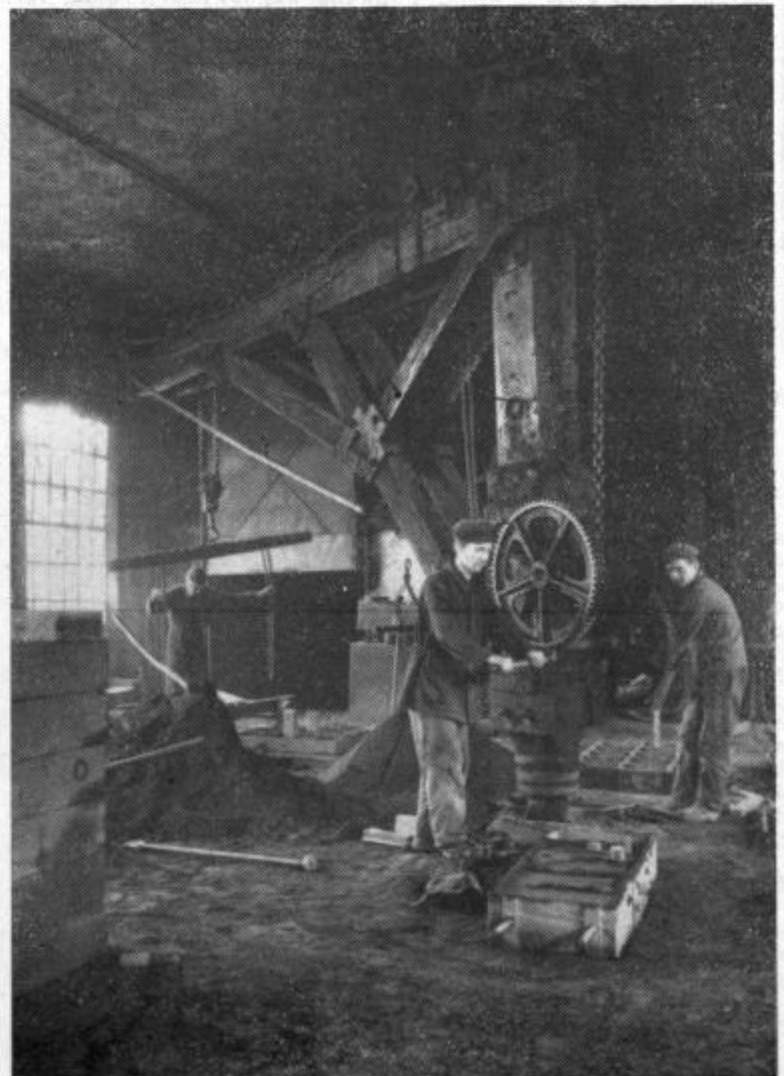
Ročno dvigalo v livarni. Konstrukcija lesena, nosilnost 2 toni, zgrajena hkrati z livarno 1900 (3)
