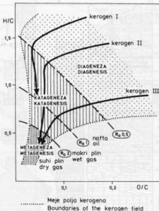
Sl. 3. Van Krevelenov diagram klasifikacije kerogena na osnovi atomskih razmerij H/C in O/C ter faze diageneze organske snovi. Za primerjavo so podane približne vrednosti odsevnosti vitrinita v % ( R_0 = 0,5-2 ); po Tissotu (1984)
