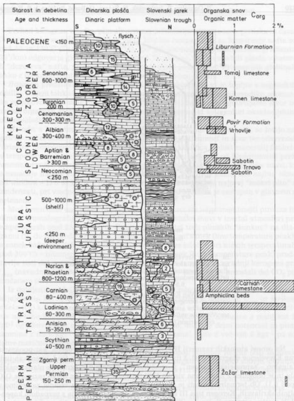
Sl. 2. Shematski litološki stolpec z raziskanimi formacijami in glavnimi geokemičnimi značilnostmi karbonatnih kamnin (delež C_{org} , indeks vitrinitne odsevnosti...). Številke v krogih pomenijo število raziskanih vzorcev posamezne formacije
