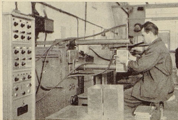
Točkasto varjenje v ročni delavnici
