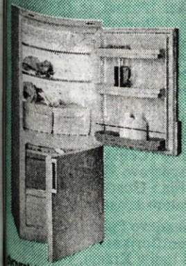
dvovratni hladilnik, IBERNA, SCM 27, skupna prostornina 268 l, hladilnik neto 173 l, zamrzovalnik neto 65 l, samodejno odvajanje, mere: 143 x 60 x 60 cm
