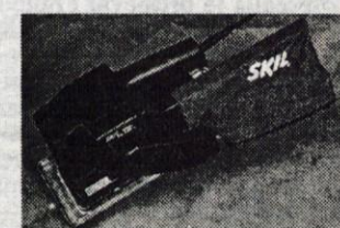
tračni brusilnik, SKIL, 1200, moč 600 W, brusna površina 76 x 130 mm
