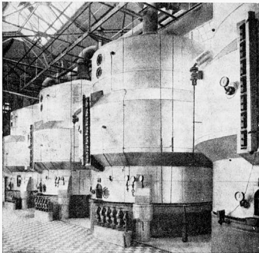
Naprave za rafiniranje sladkorja v moderni tovarni
