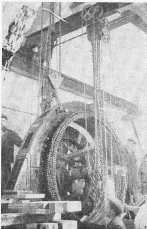
Montaža velikega jamskega kompresorja v mežiškem rudniku.
