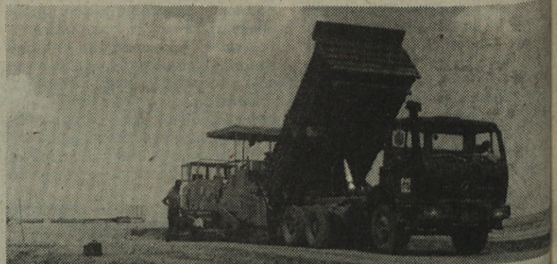
Slika je napravljena v prvih dneh aprila 1981, ko polagamo poslednje površinske cementne stabilizacije na levi obali ob nadvozu
