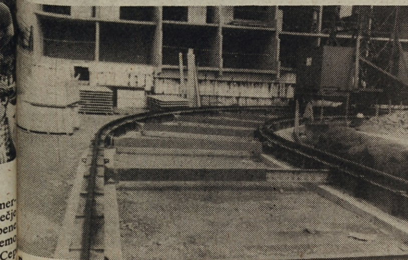
Prvič montirana žerjavna krivina za žerjav X 1266y v Mariboru na S 31, na jeklenih pajnerjih. Paziti moramo na drobni spojni material, ki se pri demontaži največkrat izgubi
