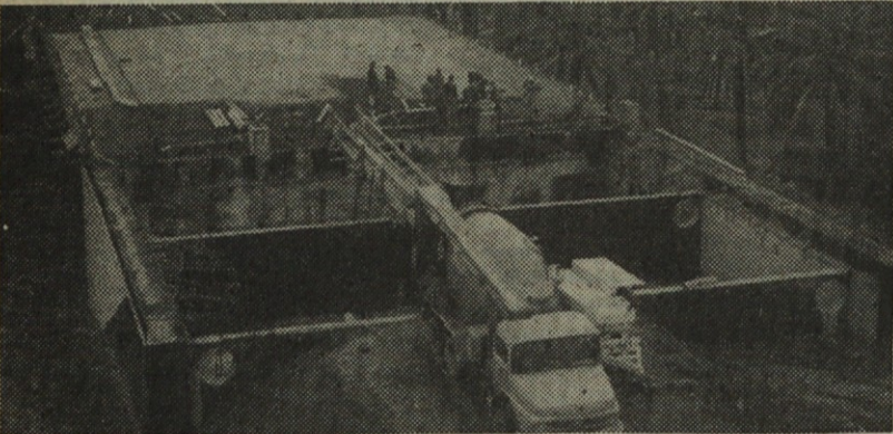
Z betoniranjem plošče na mostu preko Tigrisa smo pričeli v decembru lanskega leta. Betonirali smo po odsekih, ki so predpisani v projektu. Slikano je 20. decembra 1980
