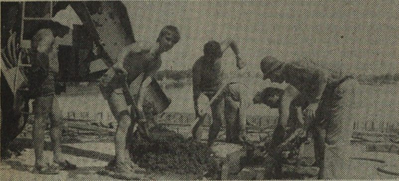
Na sliki je vgrajevanje betona ob dilataciji Maurer D-161. Dne 7. aprila 1981 so bile vgrajene vse dilatacije, zasuti Obrežni oporniki in pričeli smo s transportom preko mostu
