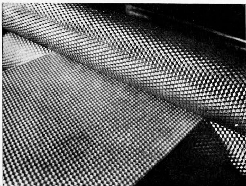
Izdelovanje satnic z valjarji
