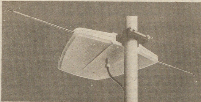
NOVA VRSTA ANTEN — V Gorenju Elrad so začeli izdelovati novo vrsto anten TVA 2002 karavan. Je univerzalna antena za sprejem TV in radijskih FM signalov. Zahvaljujoč novi tehnologiji in uporabi hibridnih vezij omogoča antena optimalni sprejem vseh signalov ob zelo majhnih dimenzijah antene. Namenjena je predvsem za montažo na bivalne avtomobilske prikolice, počitniške hišice in plovila.
