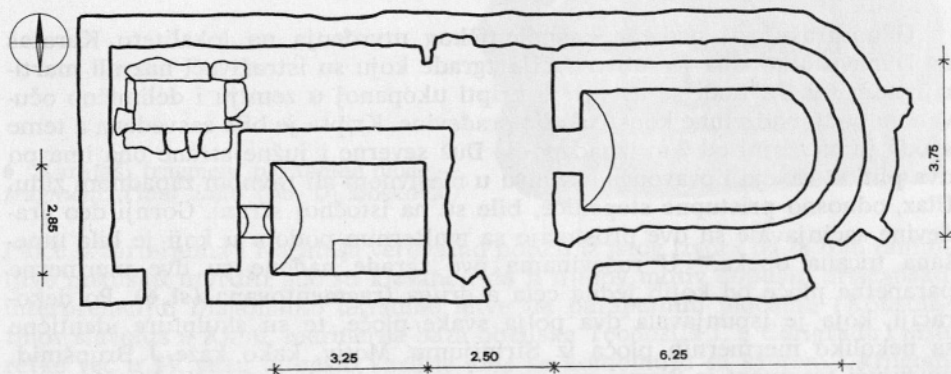
3 Crkva u Banjici kod Peći — église à Banjica près de Peć
