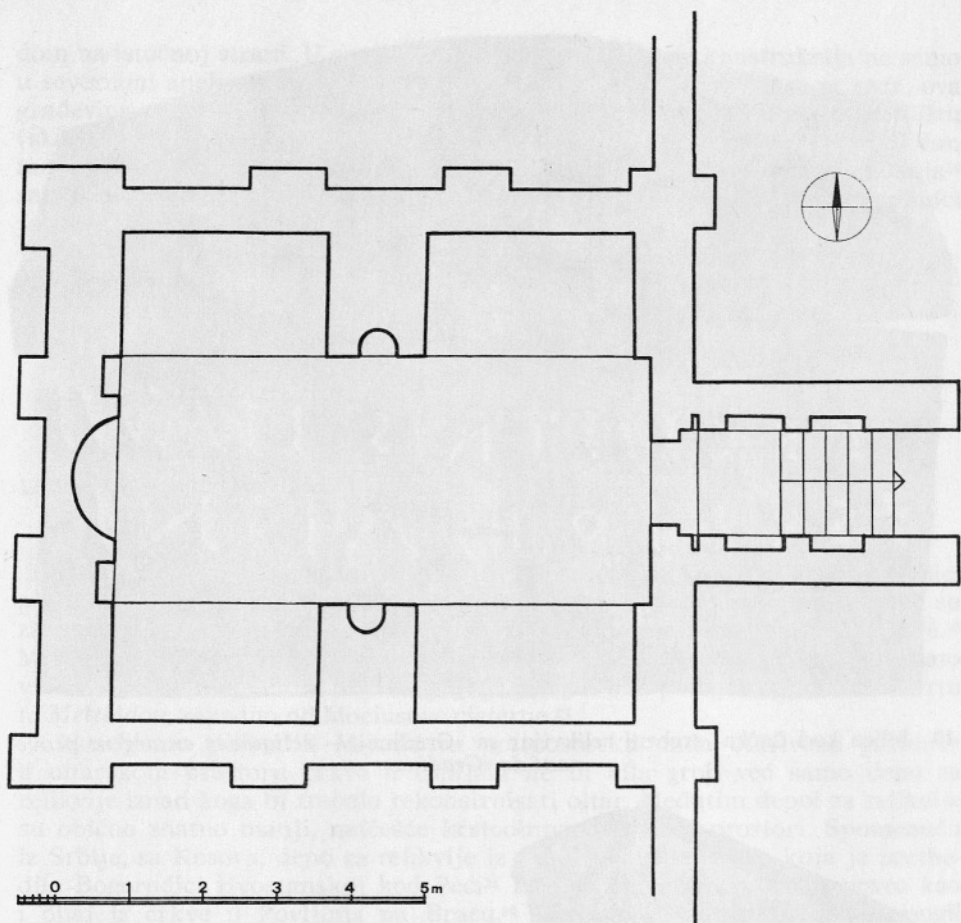
8 Niš: kripta, monumentalna grobnica — édifice funéraire (rel. N. Spremo-Petrović)
