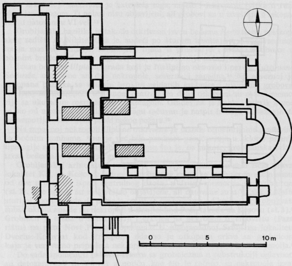
4 Caričin Grad: crkva južno od akropolja — église au sud de l'acropole
