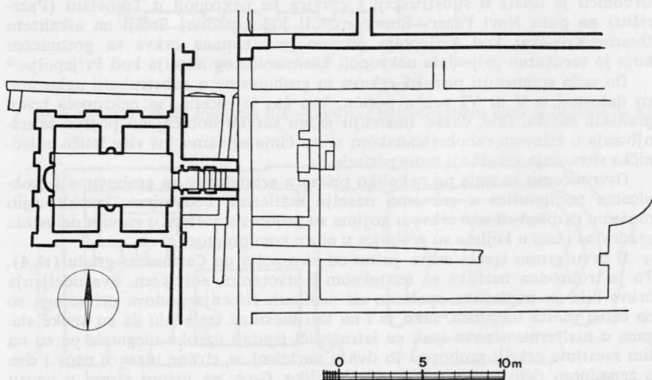
1 Niš, Jagodin Mala: ranohrišćanska crkva sa grobnicom na zapadnoj strani — église paléochrétienne avec un édifice funéraire du côté ouest (rel. N. Spremo-Petrović)
