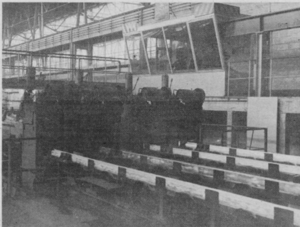
Ulivanje jeklenih gredic na napravi za kontinuirano ulivanje.
