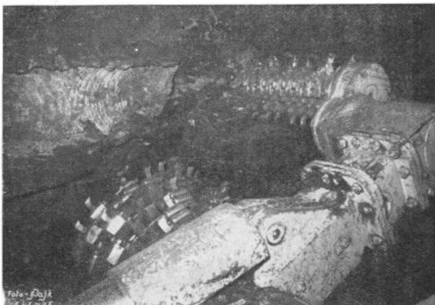
Dobivalno-nakladalni stroj »Eickhoff«
