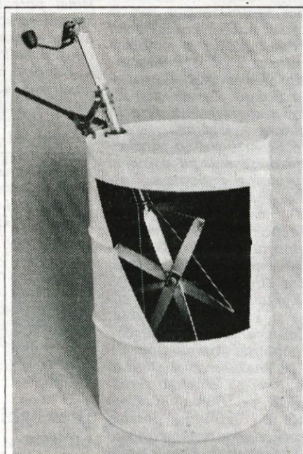
Prototip stroja na ročni pogon za mešanje tekočih kemikalij v zaprti pločevinasti posodi.
