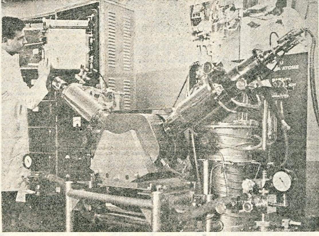
Spektrometer, skonstruiran in izdelan v Institutu »Boris Kidrič« v Vinči razbije atome in molekule različnih tež. Z njimi se s pomočjo neutronov dobivajo izotopi Urana 235. Ta spektrometer je razstavljen na Sejmu tehnike v Beogradu, ki bo trajal še do 2. septembra
