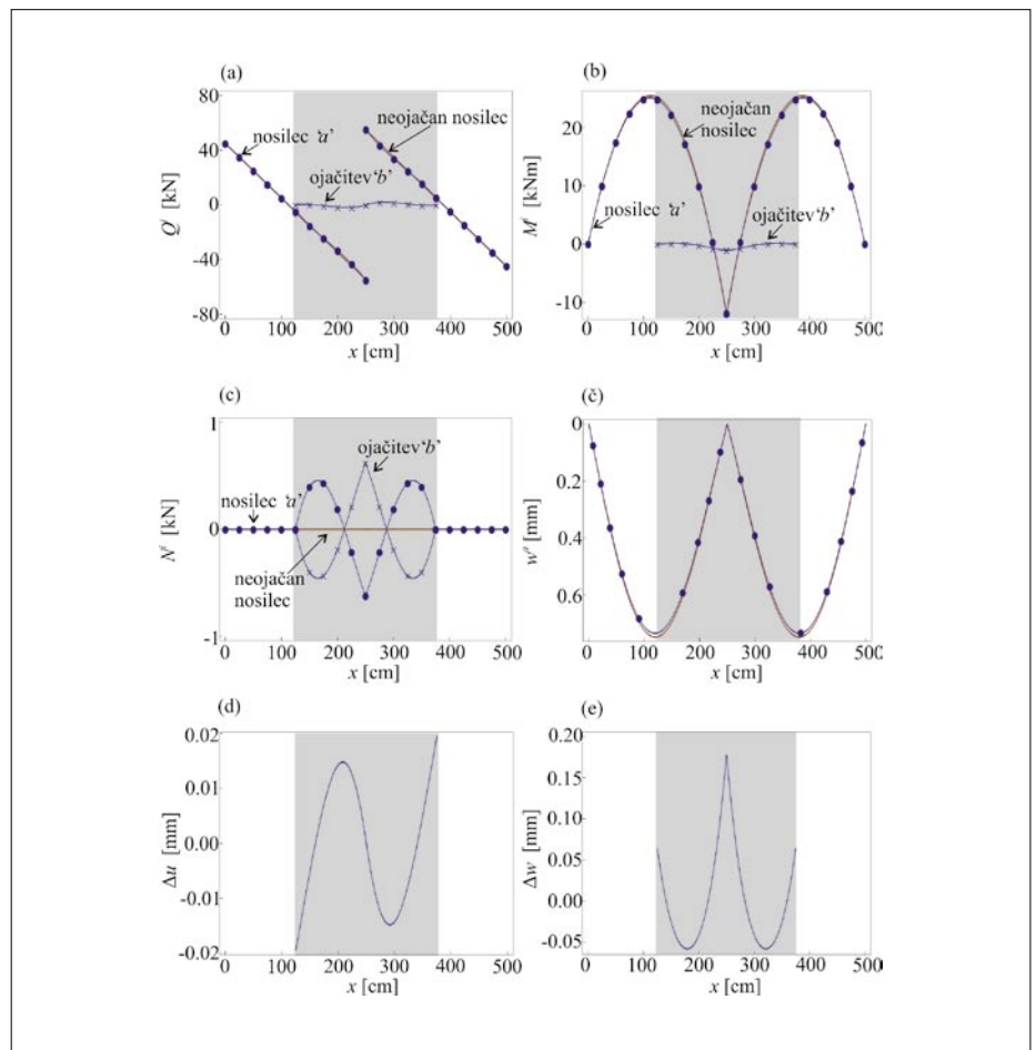
Slika 13 • Bočno ojačani razpokani kontinuirni nosilec. Primerjava med značilnimi statičnimi in kinematičnimi količinami ojačanega nosilca (modre krivulje) in neojačanega nosilca (rdeče krivulje): (a) prečne sile, (b) upogibni momenti, (c) osne sile, (č) navpični pomiki, (d) vzdolžni zamiki, (e) prečni zamiki ( k_x = k_z = 0,25 \text{ kN/cm}^3 , k_\varphi = 8,0 \cdot 10^5 \text{ kNcm} )
