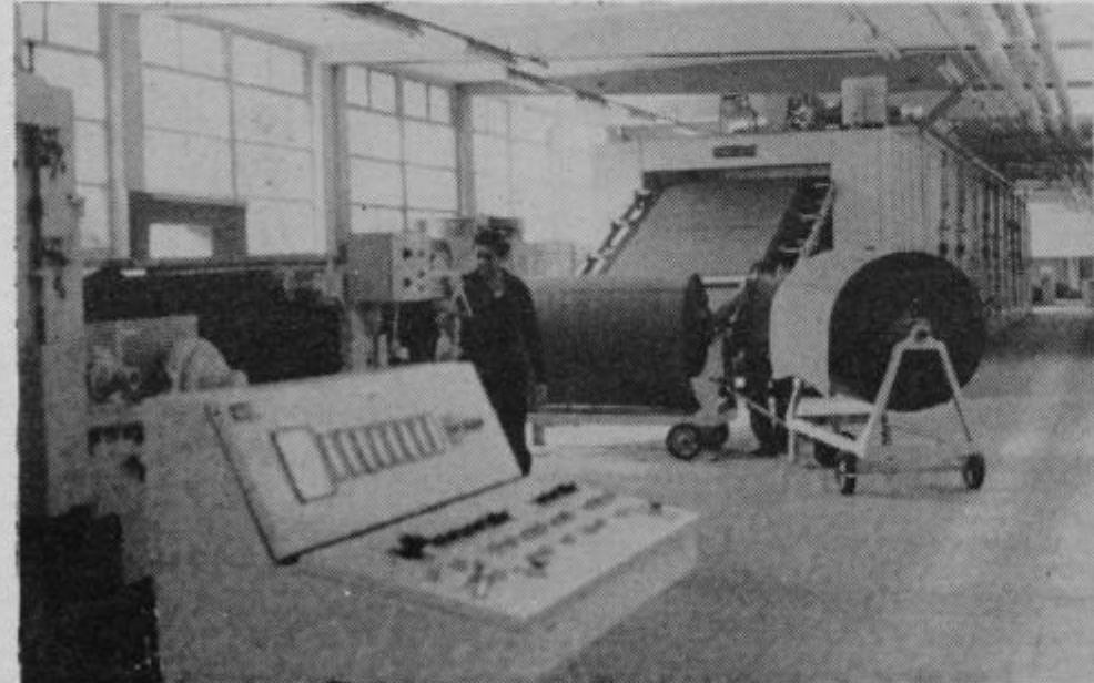
Stroj za formiranje Konita v TOZD Umetno usnje.
