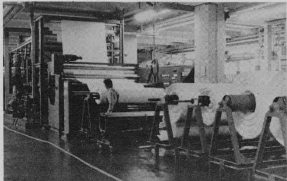
Proizvodnja netkanih materialov v TOZD Tehnična konfekcija.
