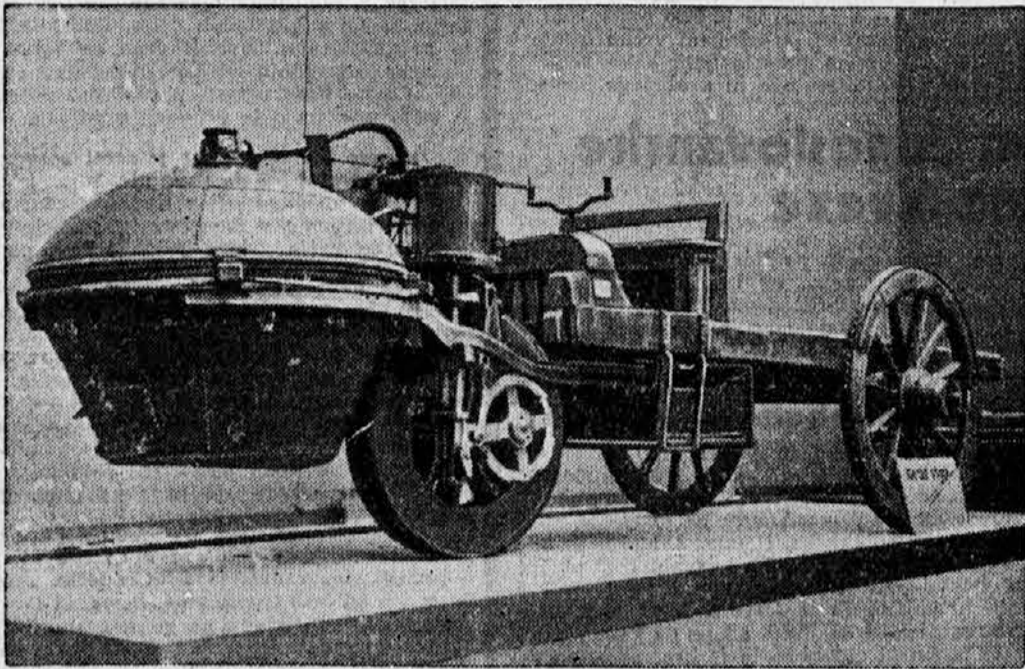
Najstarejši francoski avtomobil na sedanjih pariških razstavi. Sestavljen je leta 1771 inž. Cugnot.
