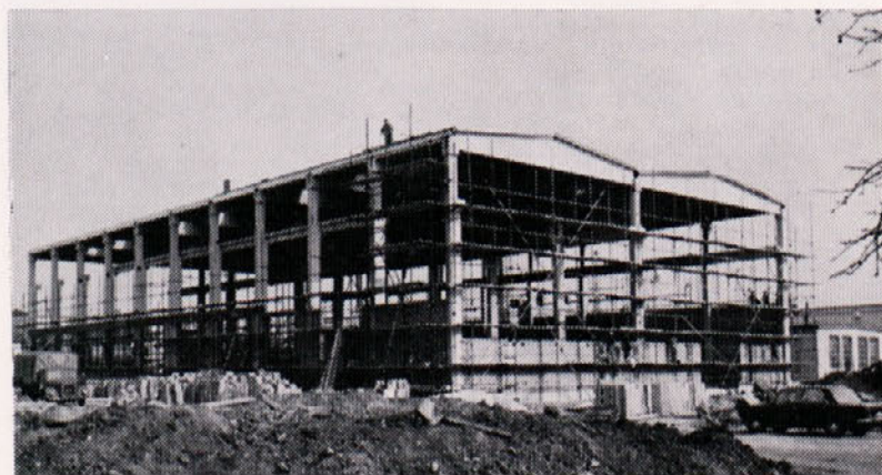
Dela na hali »Mehanizacija« izvaja TOZD GO Sentjur
