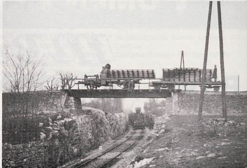
Nadvoz vojaške proge pri Krepljah.
