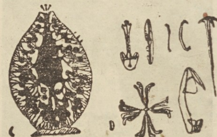
C. Shematski prerez gobe s sistemom ka nalov — D. Skeletne iglice različnih oblik
