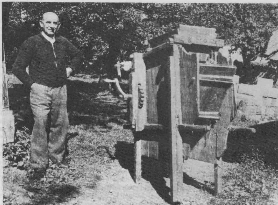
Sl. 20. Vetrnik, "vintovec". Z letnico 1803. Melviče, Ziljska dolina. Fotografiran sredi 20. stol. (J. Šušteršič. I. 1951). Lastnik negativa J. Šušteršič, Ljubljana, Igriška 6.
