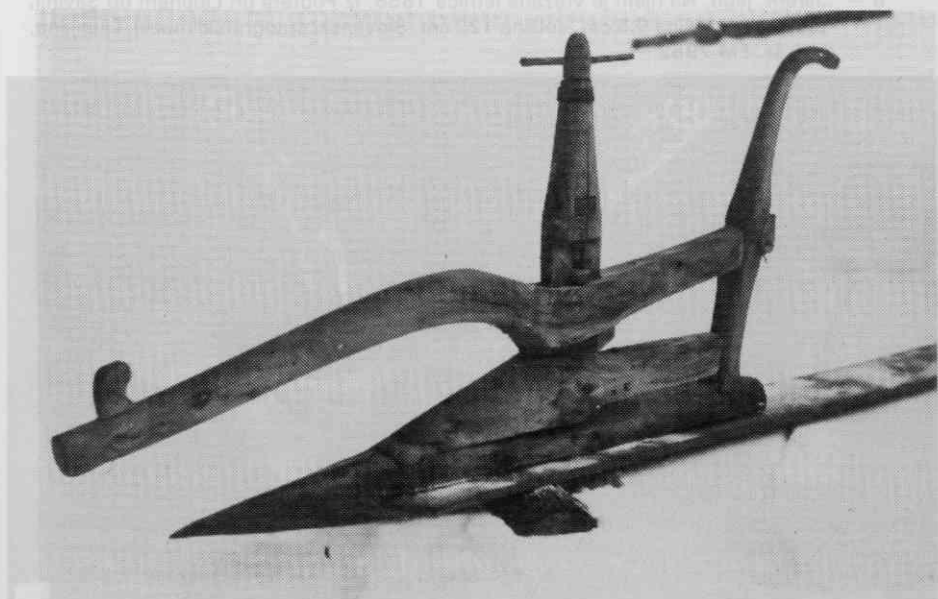
Sl. 6. Ralo iz Podvolovljeka pri Lučah. Z njim so orali še nekaj let po prvi svetovni vojni. 170 cm dolg "gredal", 82 cm visok "kôzalc", 115 cm dolg "oplas" ter 44 cm dolg in 27 cm širok lemež "raunek". Slovenski etnografski muzej, Ljubljana, inv. št. EM 7800.
