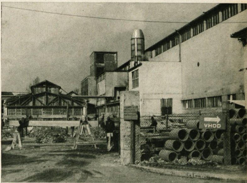
V Papirnici Količevo so v polnem teku gradbena dela rekonstrukcije kartonskega stroja KS II. Z rekonstrukcijo se bo proizvodnja kartona povečala od sedanjih 40 ton na 60 ton dnevno.
