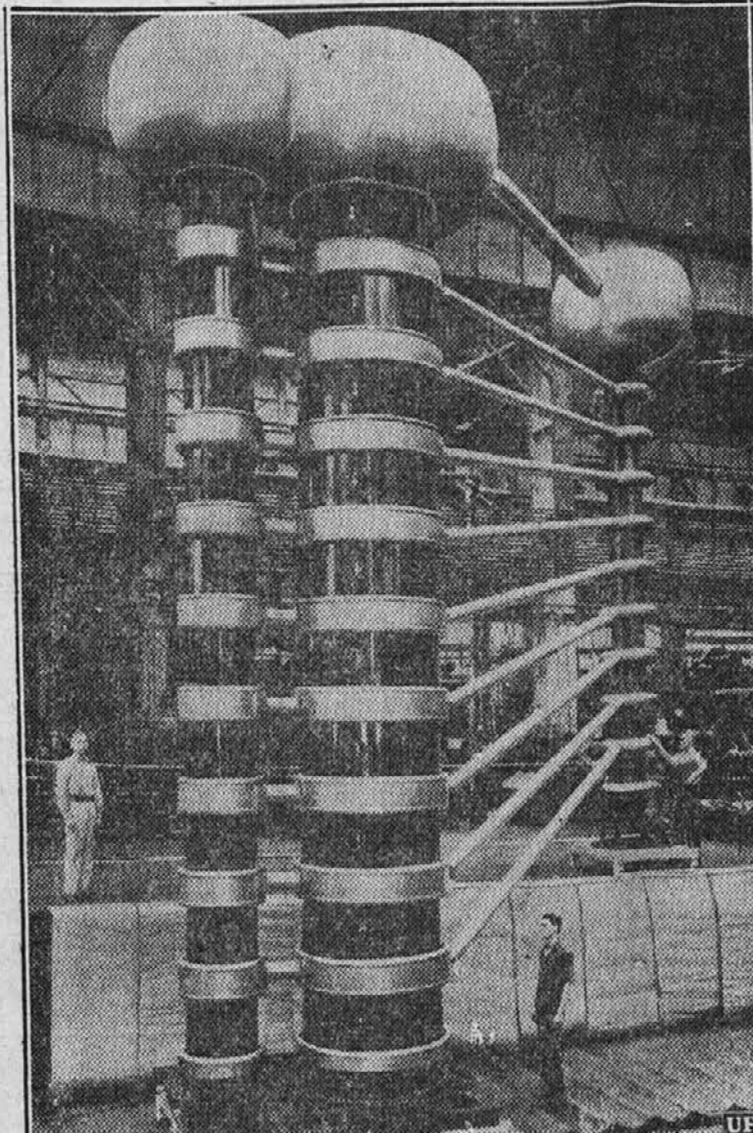
Velikanski stroj, ki proizvaja Roentgenove žarke (X-Rays), močne 1,400,000 voltov. Ta stroj je največji svoje vrste je bil izdelan v General Electric v Schenectady, N. Y., za neki federalni urad.
