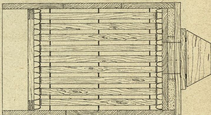
Pod. 7. Vodoravni prerez.
