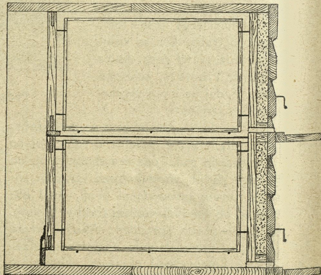
Pod. 6. Podolžni prerez.
