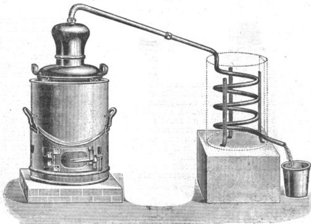
Slika 44. Brzoparilnik za žganjekuho.
