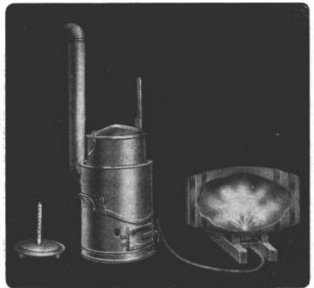
Slika 43. Brzoparilnik za preparjenje sodov.
