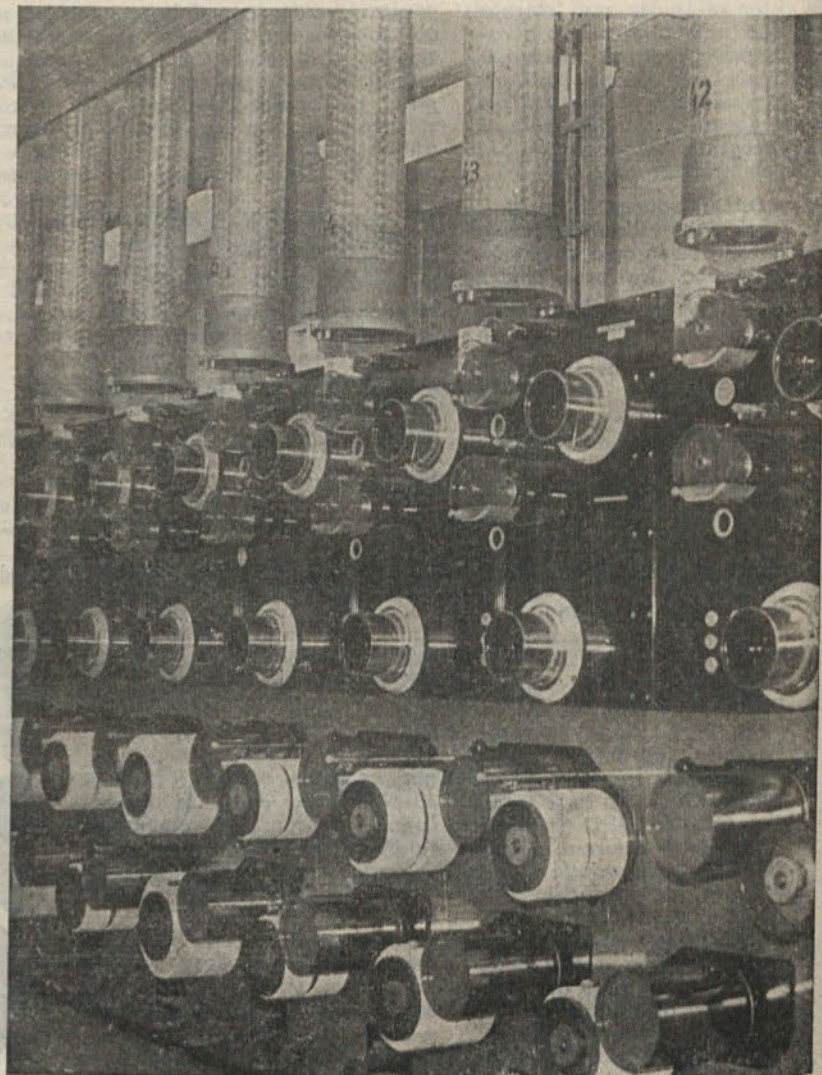
Navijalni stroj s prvim navitjem yulonskih nitk
