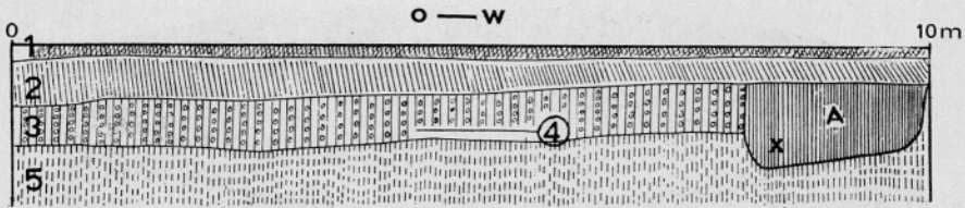
Sl. 1. Prerez slojev ob južni steni pritlične veže v Mestni hiši v Kranju (sedaj Gorenjski muzej): 1. tlak iz betona, 2. izravnalni sloj — nasutje, 3. sloj rjavega humusa s prodrom in staroslovanskimi skeletnimi grobovi, 4. staroslovanski skelet moškega (št. 4) v globini 0,90 m s pridatkom bronastega obsenčnega obročka z S zanko in kvačico ob levi senčnici, 5. prod — sterilni sloj, A — odpadna jama in mesto najdbe (X) opisanih delov keramičnih posod
