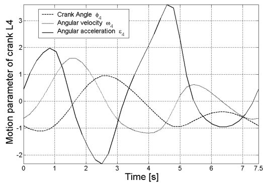
Fig. 5. Motion parameter of crank L_4
