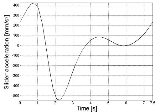
Fig. 4. Slider acceleration \ddot{S}
