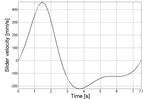
Fig. 3. Slider velocity \dot{S}
