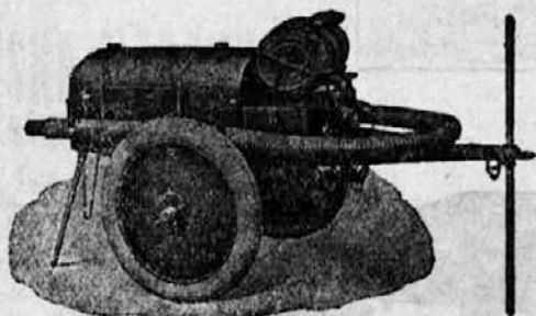
Lahka, dvokolna motorna brizgalnica z 16/18 HP motorjem, dobava vode 800 l v minuti, pritisk do 12 atm.
