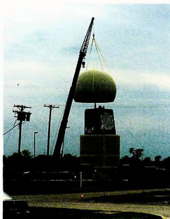
Tornade odkriva Dopplerjev radar.
