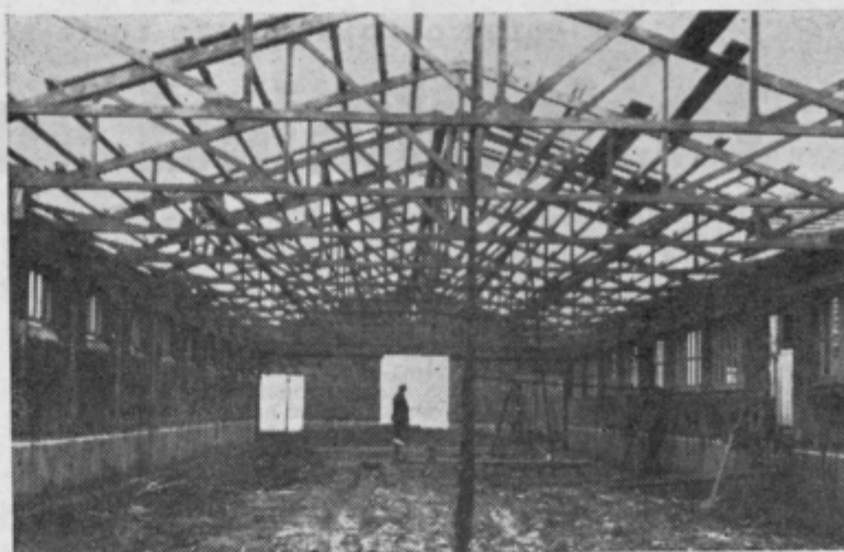
Železna konstrukcija sodobnega hleva za 100 glav goveje živine, ki ga gradijo v Podlogu. Za mlečno farmo v Podlogu bodo zgradili štiri take hleve.
