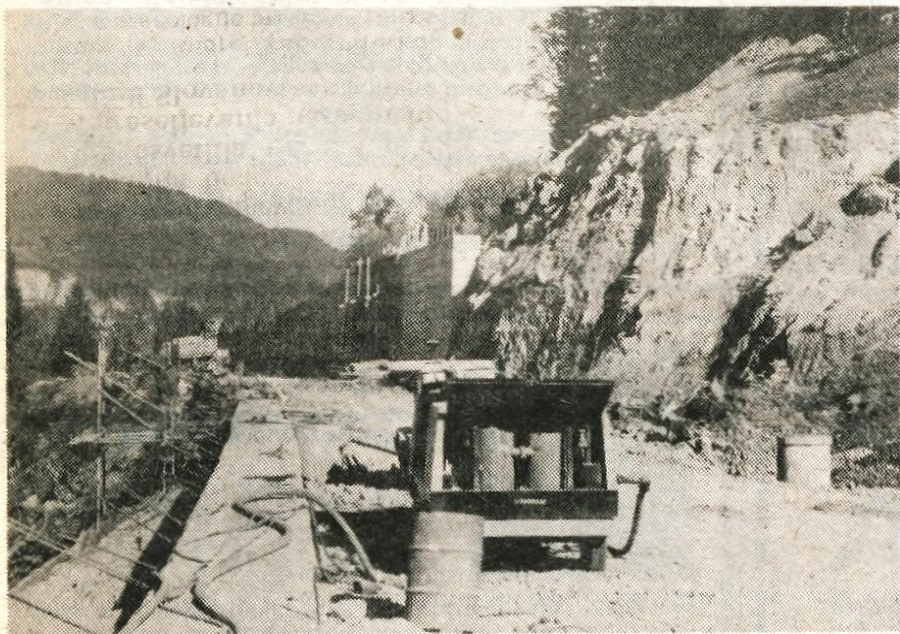
Na najzahtevnejšem, 120 metrov dolgem odseku, kjer je bilo treba »presekati« aktivni zemeljski plaz in na zgornjem ter spodnjem delu ceste zgraditi pilotni steni, poteka še zadnji izkop. V piloti in steno je bilo vgrajenega 1800 kubičnih metrov betona. Na celotni trasi pa je bilo izkopenega in vgrajenega 140.000 kubičnih metrov materiala.
