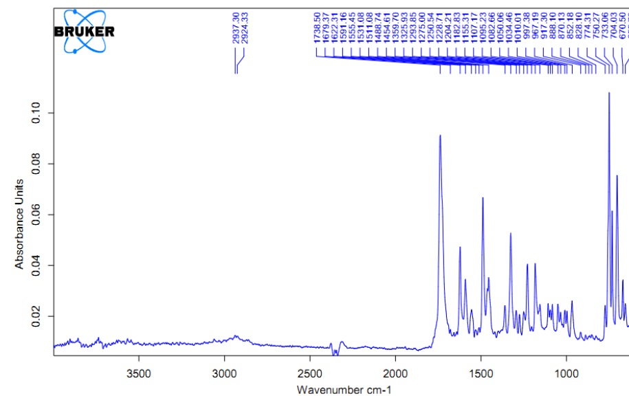
Substance 2.4 IR spectrum
