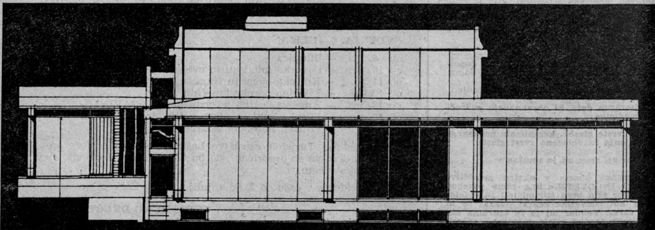
STRANSKI DEL BODOČE PREDELOVALNICE MESA KMETIJSKE ZADRUGE V LAŠKEM
