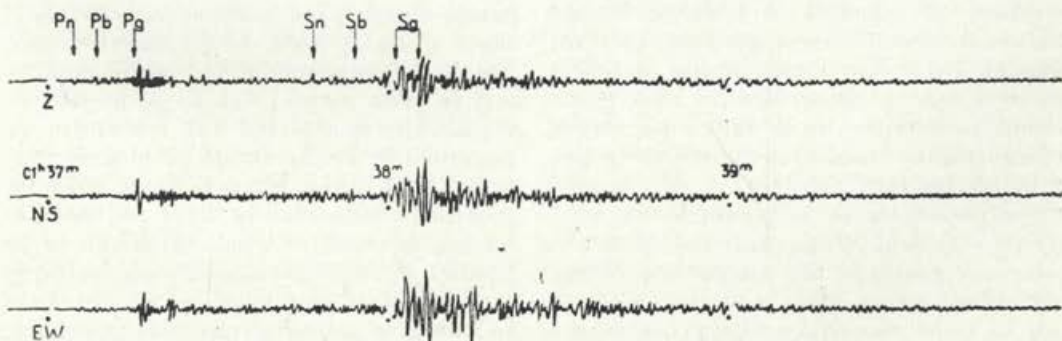
Seizmogram bližnjega potresa, registriranega s tremi kratko-periodičnimi seizmografi po Hillerju, tipa »Stuttgart«. — Epicenter: Gornja Italija, razdalja 380 kilometrov, azimut SE Registrirano v Stuttgartu 18. I. 1952
