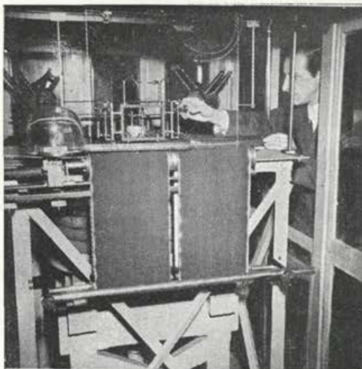
Wiechertov astatični horizontalni seizmograf (za registracijo horizontalnih premikov zemlje). Masa = 1.000 kg
