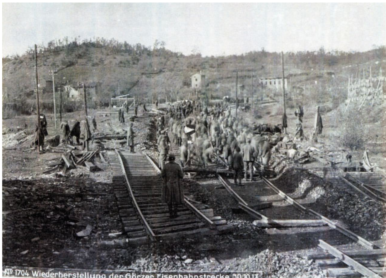
Slika 7 Obnovitvena dela na progi med Šempetrom pri Gorici in Volčjo Drago konec oktobra 1917 (vir Splet 11).
