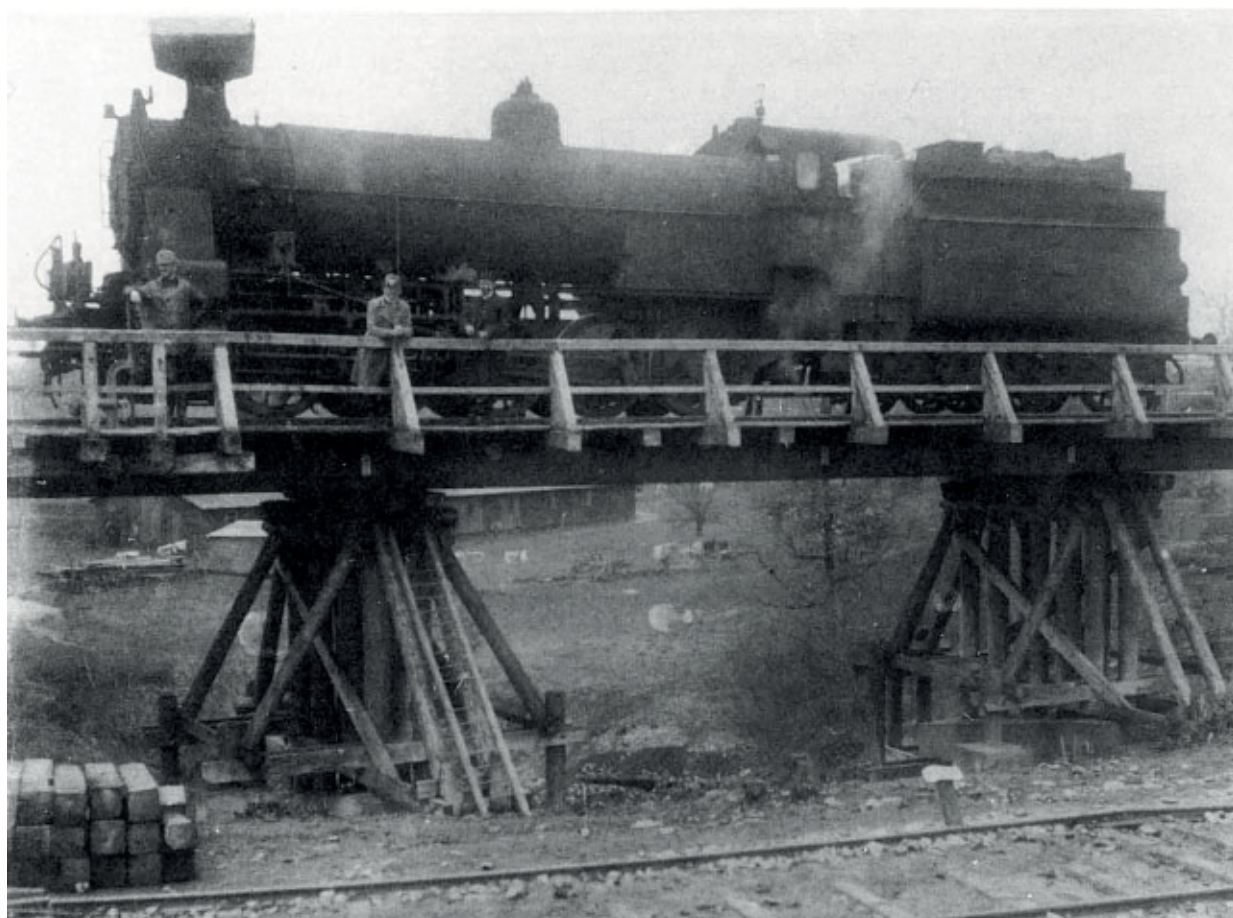
Slika 119 Eden izmed treh mostov obvozne trase (po Schaumann 1991, 157).
