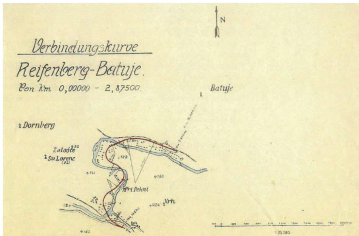
Slika 118 2,875 kilometra dolg zvezni lok skozi sotesko Pekel, ki je povezal železniški progj Jesenice–Trst in Gorica–Ajdovščina (po Rustja 2002, 84).
