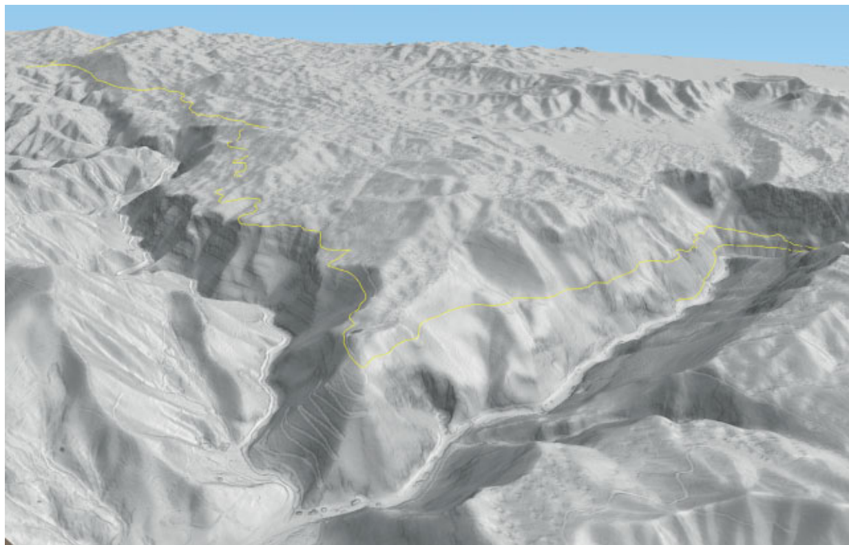
Slika 163 3D-prikaz lidarskega posnetka: pogled proti jugu na traso nekdanje železnice Godovič–Idrija (kat. št. 276) (izvedba M. Mori).
