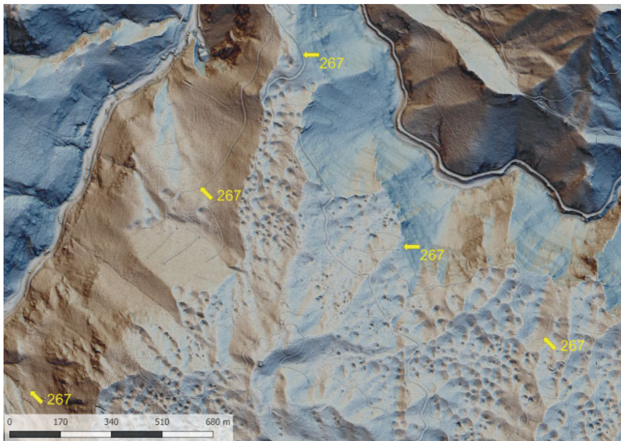
Slika 162 Lidarski posnetek: trasa nekdanje železnice Godovič–Idrija (kat. št. 267) (izvedba M. Mori).
