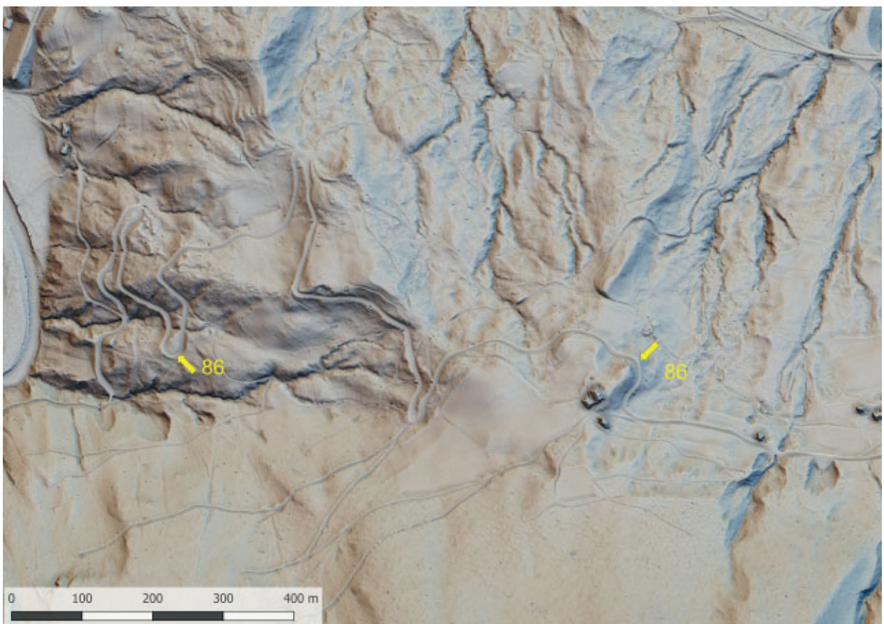
Slika 74 Lidarski posnetek: cesta Grabovo–Bukovo–Reka, odsek vzhodno od Grabovega (kat. št. 86) (izvedba M. Mori).
