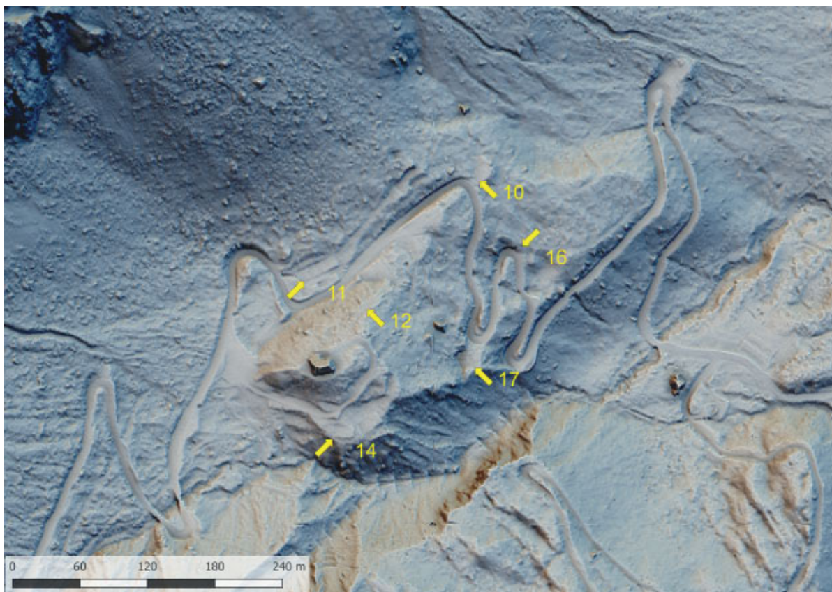
Slika 15 Lidarski posnetek: ruska cesta na Vršič (kat. št. 16), lokacija grobišča ruskih vojnih ujetnikov pod Erjavčovo kočo (kat. št. 12), terasa vmesne postaje žičnice in severnega taborišča (kat. št. 17 in 14), terasa taboriščne ambulante (kat. št. 10) ter ostanki taboriščne kuhinje, pekarnice in konjušnice (kat. št. 11) (izvedba M. Mori).
