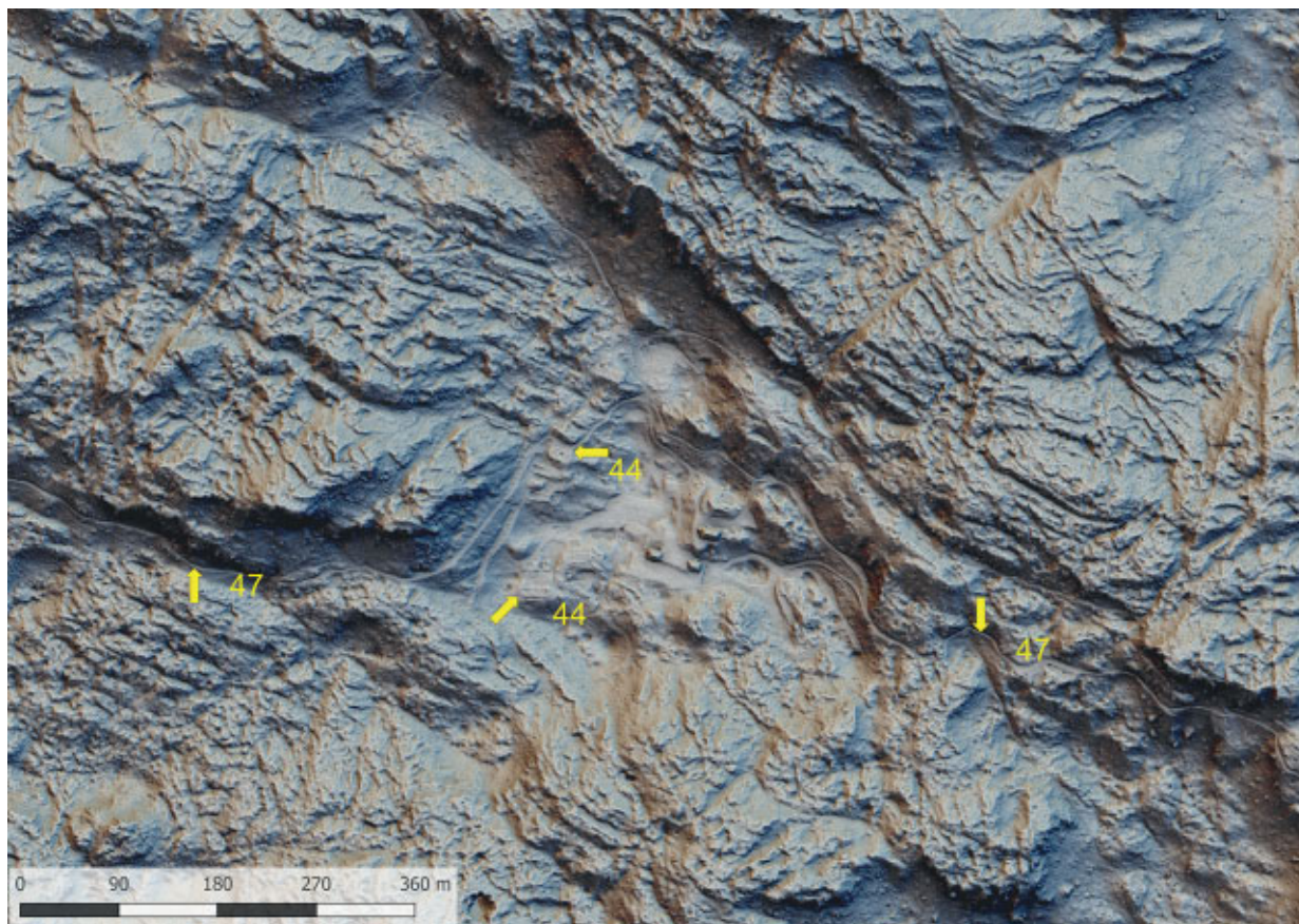
Slika 31 Lidarski posnetek: ostanki stavb taborišča na Planini na Kraju (kat. št. 44) ter odsek poti Savica–Bogatinsko sedlo–Peski–Duplje (kat. št. 47) (izvedba M. Mori).
