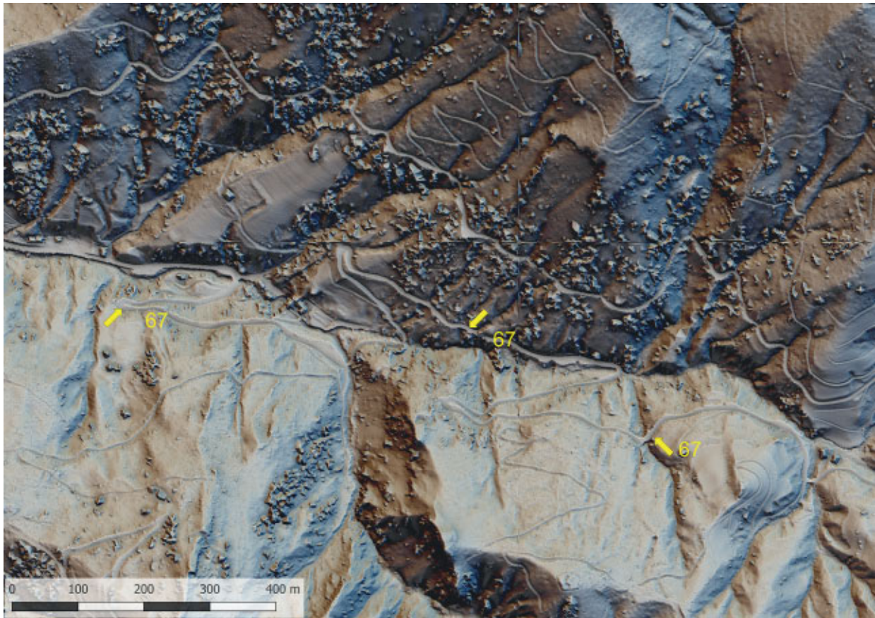
Slika 60 Lidarski posnetek: srednji odsek ceste Podbrdo–Petrovo brdo (kat. št. 67) (izvedba M. Mori).
