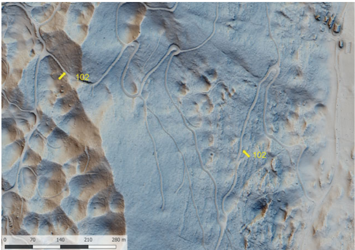
Slika 80 Lidarski posnetek: cesta Občina–Gornji Lokovec (kat. št. 102) (izvedba M. Mori).
