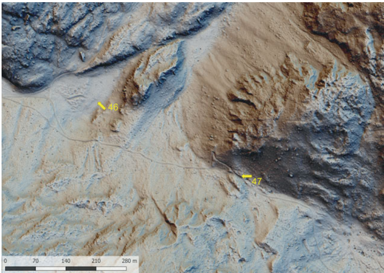
Slika 34 Lidarski posnetek: približna lokacija pokopa treh ruskih vojakov (kat. št. 46) ter odsek poti Savica–Bogatinsko sedlo–Peski–Duple na planini Duple (kat. št. 47) (izvedba M. Mori).
