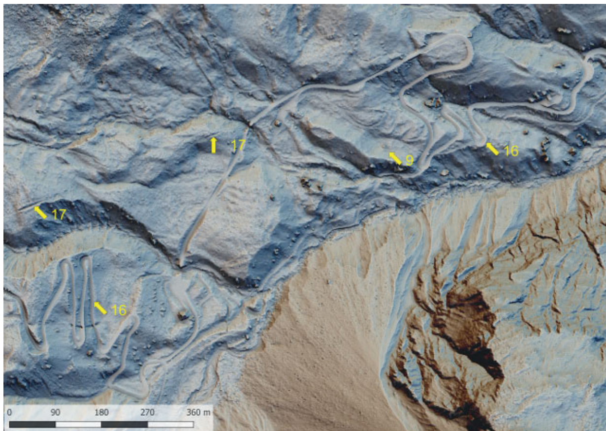
Slika 7 Lidarski posnetek: Rуска kapelica (kat. št. 9), nseki za žičnico (kat. št. 17) ter ruska cesta na Vršič (kat. št. 16) (izvedba M. Mori).
