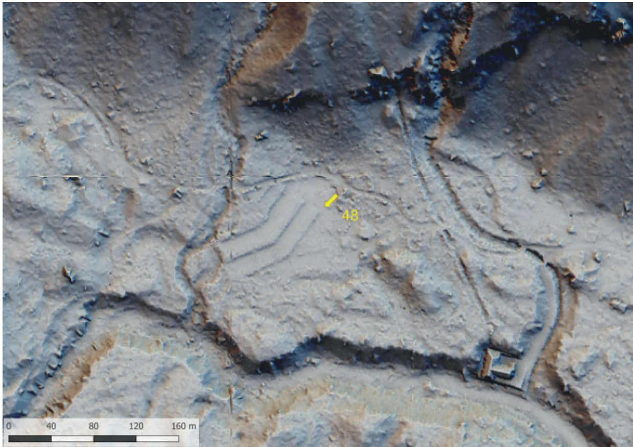
Slika 40 Lidarski posnetek: terase taborišča ruskih vojnih ujetnikov v Ukancu (kat. št. 48) (izvedba M. Mori).
