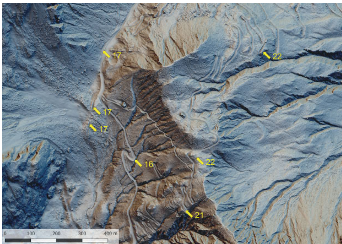
Slika 16 Lidarski posnetek: ostanki žičnice in obvozne žičnice na Vršič (kat. št. 17 in 22), ruska cesta ter obvozna cesta na Vršič (kat. št. 16 in 21) (izvedba M. Mori).
