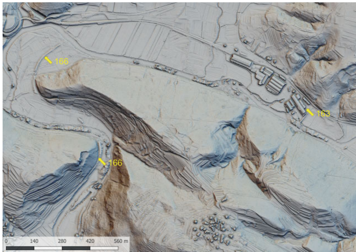
Slika 117 Lidarski posnetek: lokacija Muličeve fužine (kat. št. 163) ter ostanki nasipov in vsekov za železnico Batuje–Saksid (kat. št. 166) (izvedba M. Mori).
