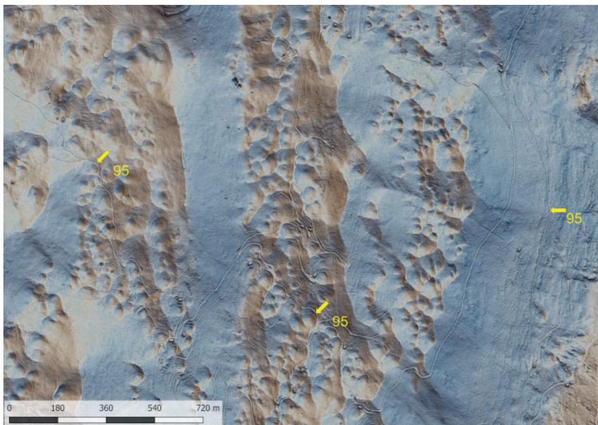
Slika 77 Lidarski posnetek: Borojevičeva cesta, odsek med Vrati in Grivo (kat. št. 95) (izvedba M. Mori).
