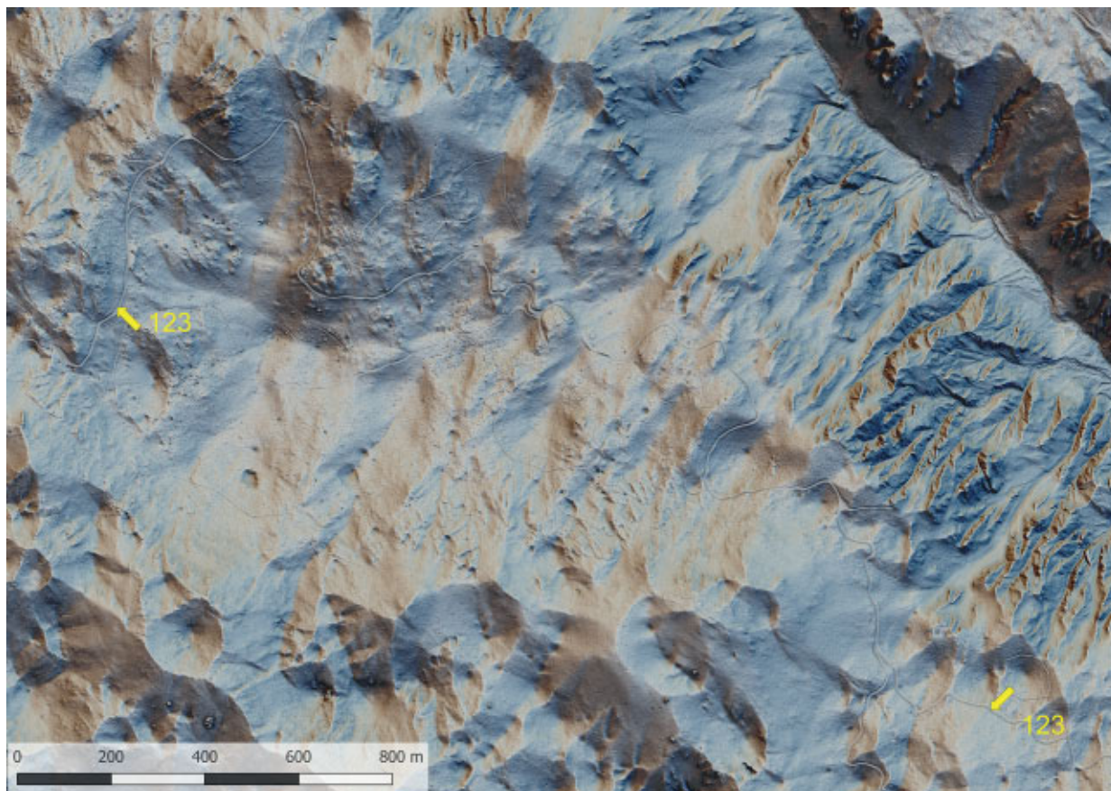
Slika 87 Lidarski posnetek: cesta Male Lazne–Mala gora, osrednji odsek (kat. št. 123) (izvedba M. Mori).
