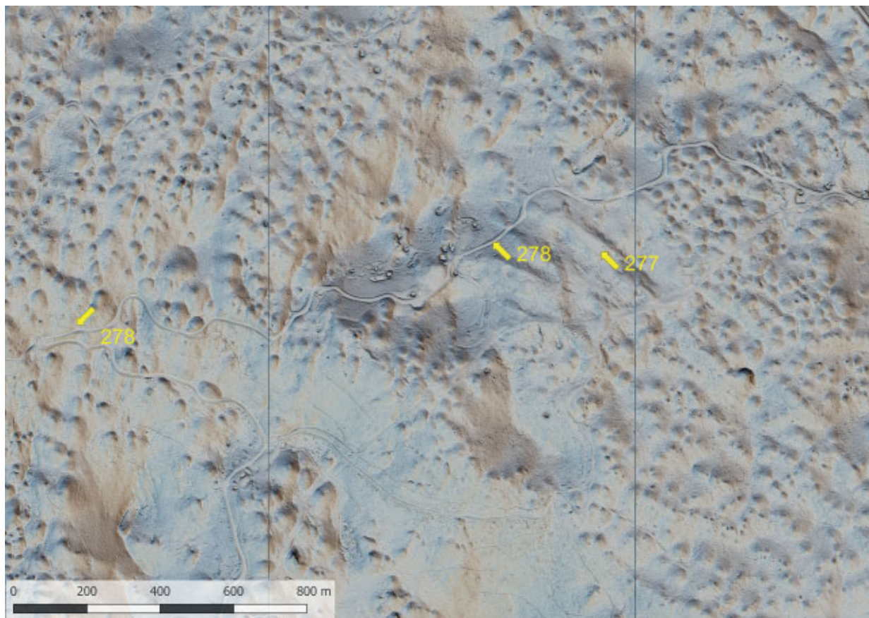
Slika 167 Lidarski posnetek: Cesta Kalce–Podkraj (kat. št. 278). Ostrega ovinka v zahodnem delu se je prijelo ime Ruska rajda. Lokacija taboriščne doline Kalce (kat. št. 277) (izvedba M. Mori).
