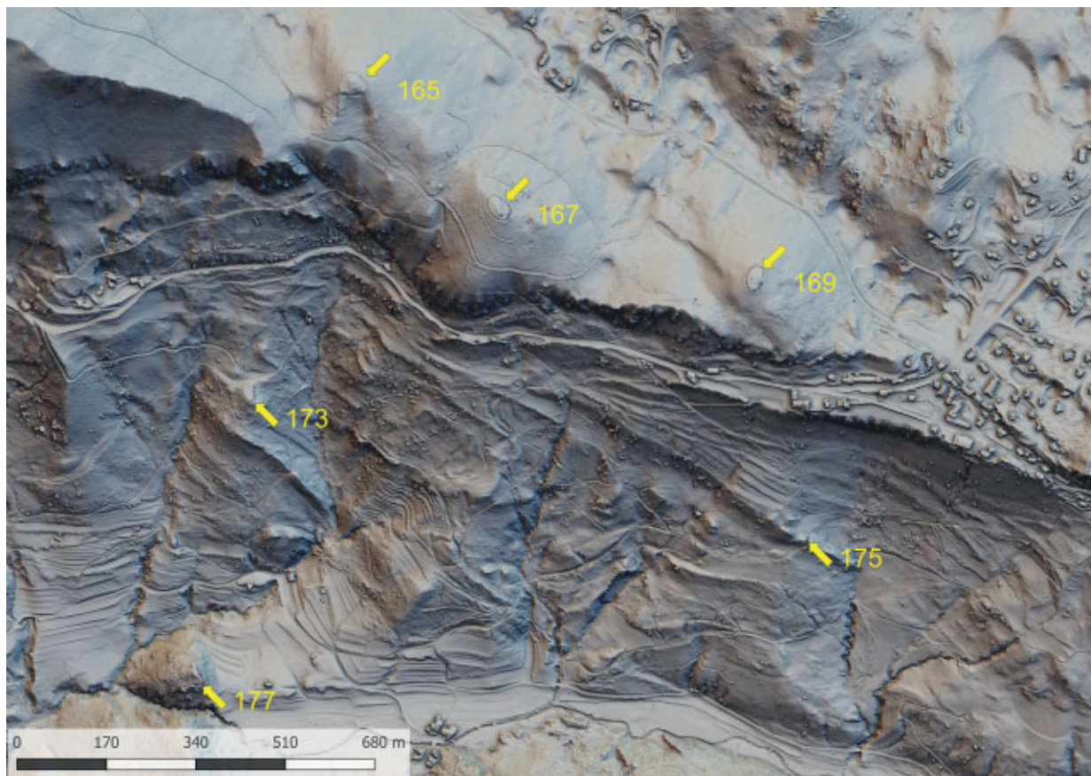
Slika 122 Lidarski posnetek: vojaški jarki na utrdbah 6 (kat. št. 177), 7 (kat. št. 173), 8 (kat. št. 165), 9 (kat. št. 167) in 10 (kat. št. 169) ter vsek Na Grebenici (kat. št. 175) (izvedba M. Mori).
