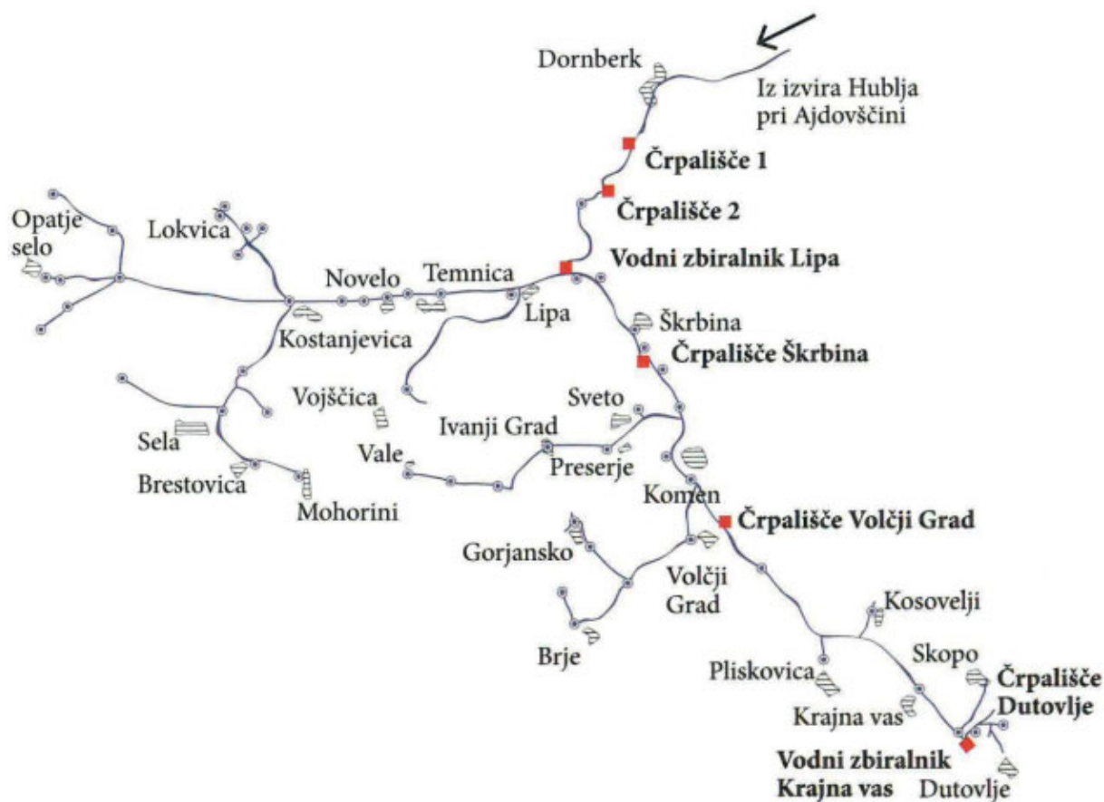
Slika 100 Vsi kraki kraškega vodovoda, glavna črpališča in zbiralniki, ki jih je napajala voda iz Hublja (po Klavora 2014a, 70).
