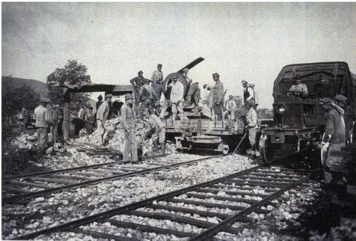
Slika 5 Izgradnja železniške postaje pri Britofu pri Povirju na Krasu (po Schaumann 1991, 171).
