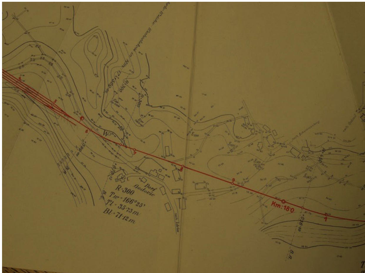
Slika 160 Načrt poteka normalnotirne proge v Godoviču z izrisanimi stavbami centra vasi leta 1917 (po Splet 31).
