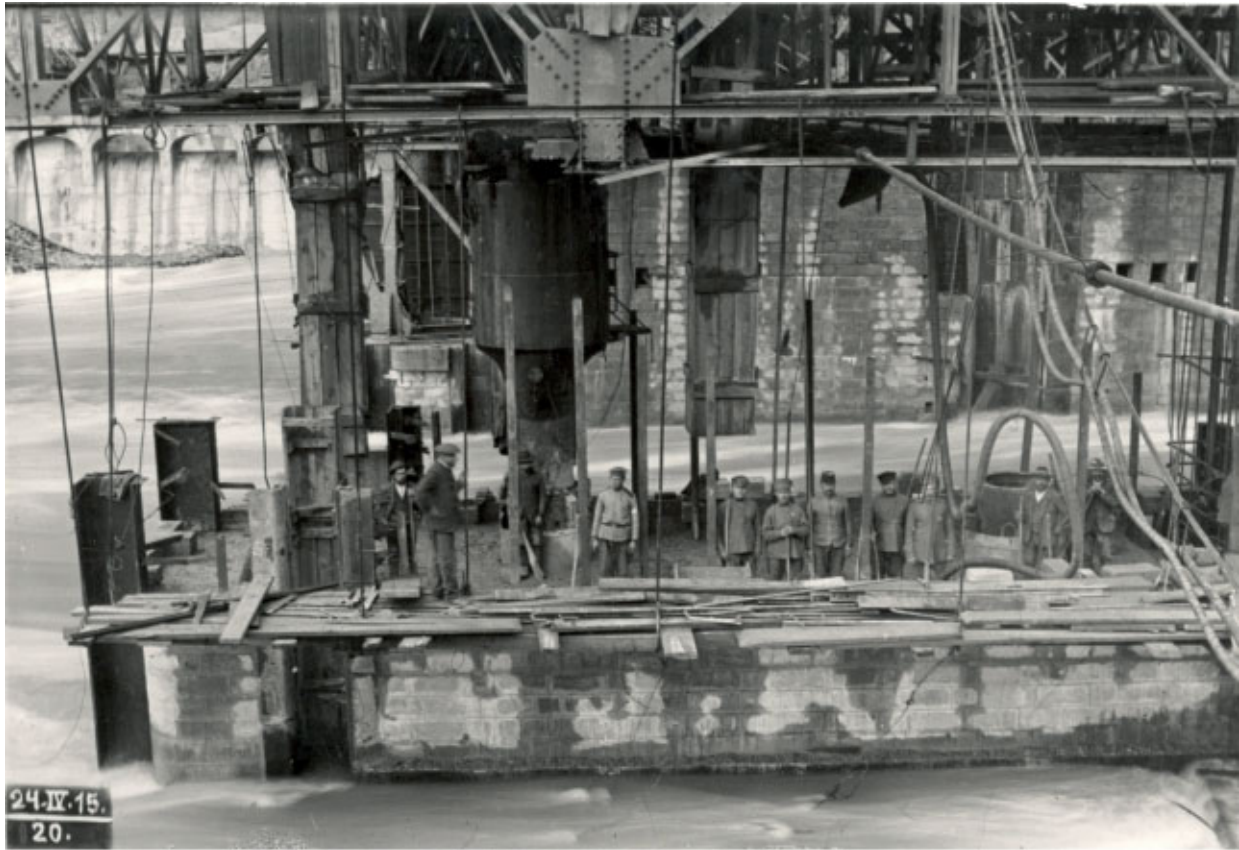
Slika 176 Gradnja HE Fala 24. aprila 1915 (po Lešnik 2017, 16).
