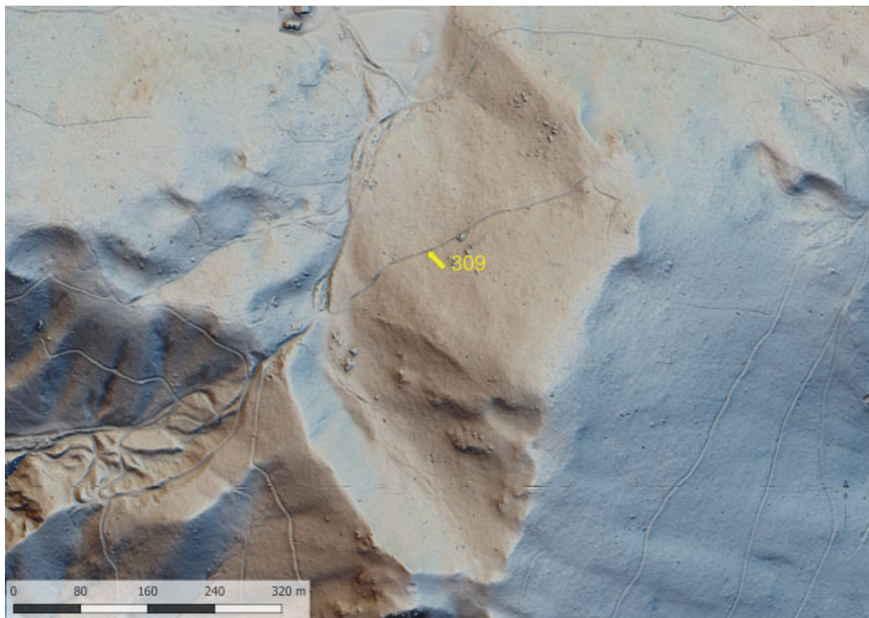
Slika 171 Lidarski posnetek: cesta na Kurnikov vrh nad Zgornjim Breznom (kat. št. 309) (izvedba M. Mori).
