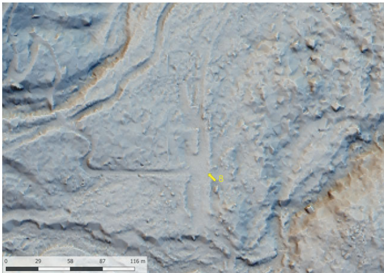
Slika 3 Lidarski posnetek terase taborišča ruskih vojnih ujetnikov pri Kranjski Gori (kat. št. 8) (izvedba M. Mori).
