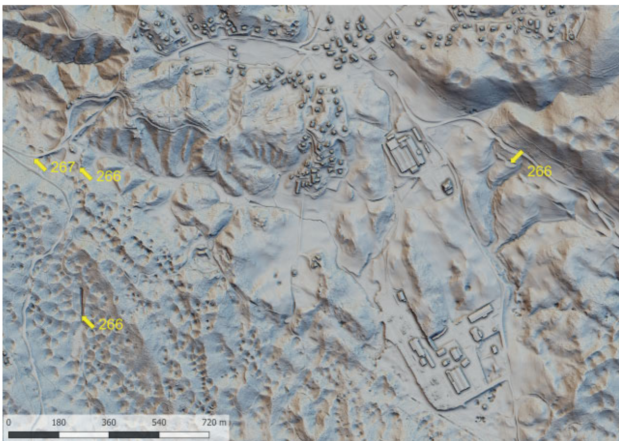
Slika 159 Lidarski posnetek: trasa nekdanje železnice Dolnji Logatec–Kalce–Hotedršica–Godovič–Črni Vrb–Zadlog–Poncala, odsek pri Godoviču (kat. št. 266) ter odcep lokalne linije Godovič–Idrija (kat. št. 267) (izvedba M. Mori).
