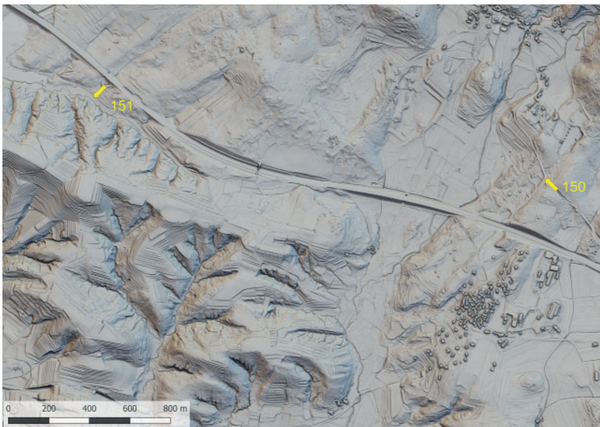
Slika 105 Lidarski posnetek: odseka cesti Batuje–Črniče (kat. št. 150) ter Batuje–Vogrsko (kat. št. 151) (izvedba M. Mori).
