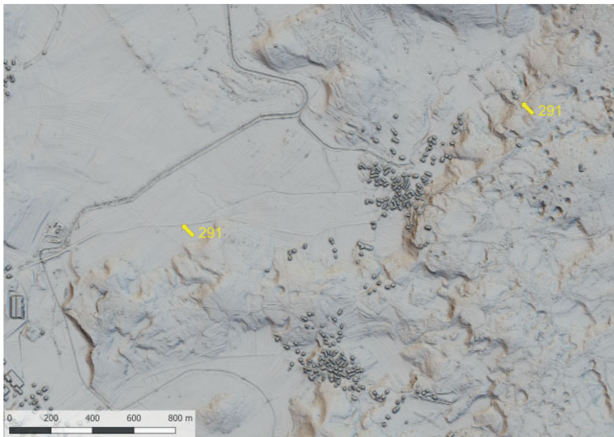
Slika 168 Lidarski posnetek: trasa nekdanje ozkotirne železnice Pivka–Javornik, odsek vzhodno od Pivke (kat. št. 291) (izvedba M. Mori).
