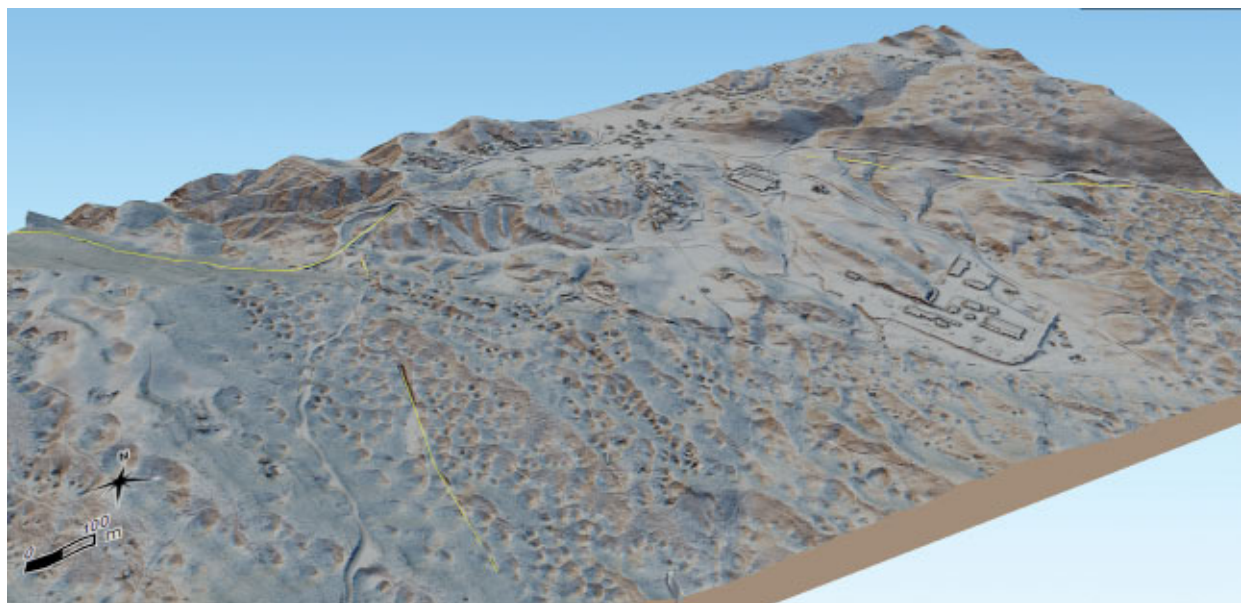
Slika 161 3D-prikaz lidarskega posnetka: pogled proti severu železniško križišče pri Godoviču (kat. št. 266 in 267) (izvedba M. Mori).
