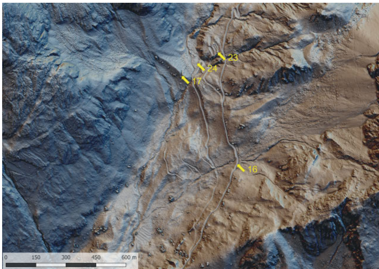
Slika 19 Lidarski posnetek: terase južnega taborišča (kat. št. 23), lokacija pokopov ujetnikov (kat. št. 24), usek za žičnico (kat. št. 17) ter ruska cesta na Vršič (kat. št. 16) (izvedba M. Mori).
