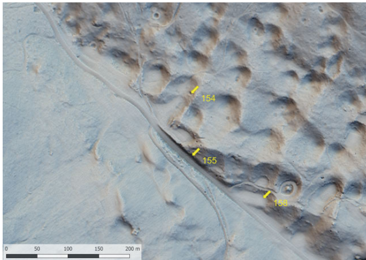
Slika 113 Lidarski posnetek: lokacija Pri ruski kuhinji (kat. št. 154), cestni vsek Ajnšnit (kat. št. 155) ter nasutje izkopanega materiala (kat. št. 158) (izvedba M. Mori).
