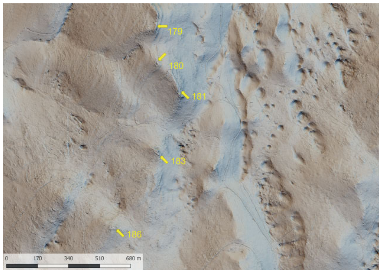
Slika 134 Lidarski posnetek: vojaški jarki na utrdbah 1 (kat. št. 186), 2 (kat. št. 183), 3 (kat. št. 181), 4 (kat. št. 180) in 5 (kat. št. 179) (izvedba M. Morj).
