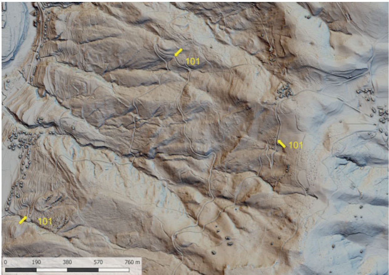
Slika 79 Lidarski posnetek: cesta Kanal–Kanalski Vrh (kat. št. 101) (izvedba M. Mori).
