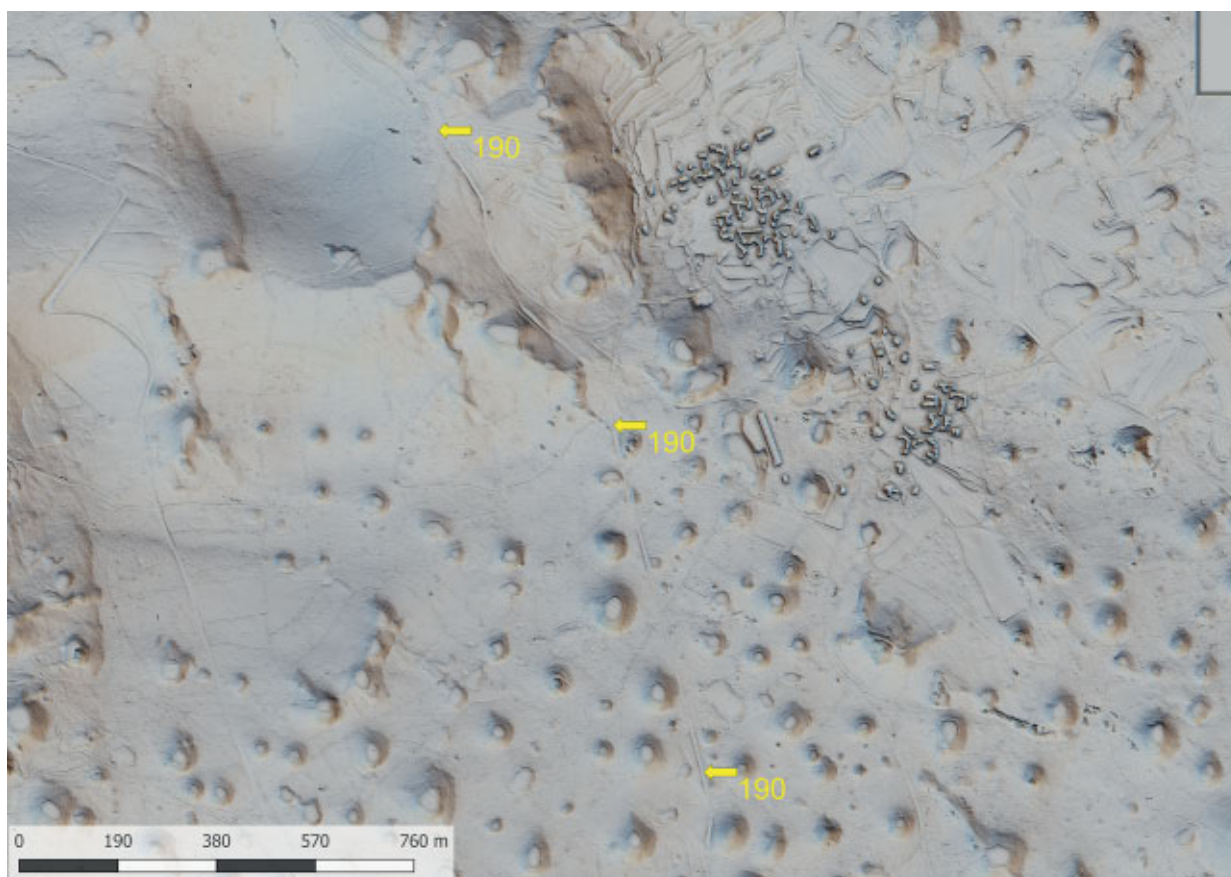
Slika 141 Lidarski posnetek: železnica Dutonje–Komen–Kostanjevica na Krasi, odsek pri Gabrovici pri Komnu (kat. št. 190) (izvedba M. Mori).
