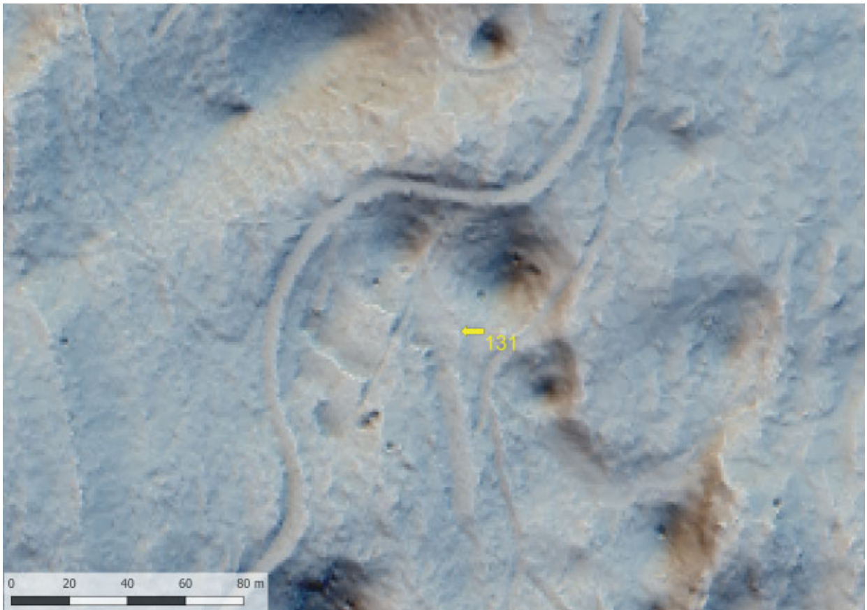
Slika 90 Lidarski posnetek: terase, na katerih so stale vojaške barake (kat. št. 131) (izvedba M. Mori).
