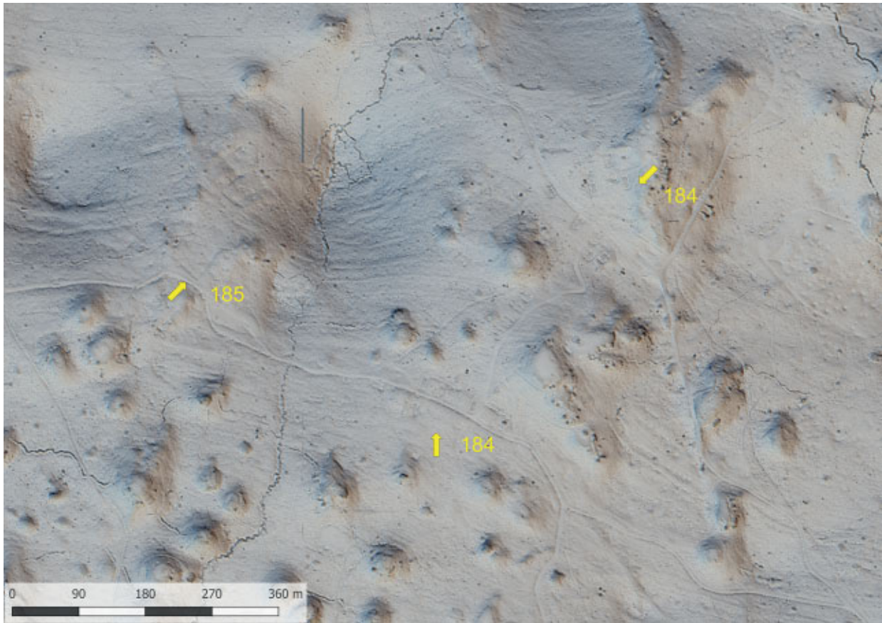
Slika 129 Liderski posnetek: sledovi stanb tabora Segeti (kat. št. 184) ter odsek ceste Kostanjevica–Lokvica (kat. št. 185) (izvedba M. Mori).
