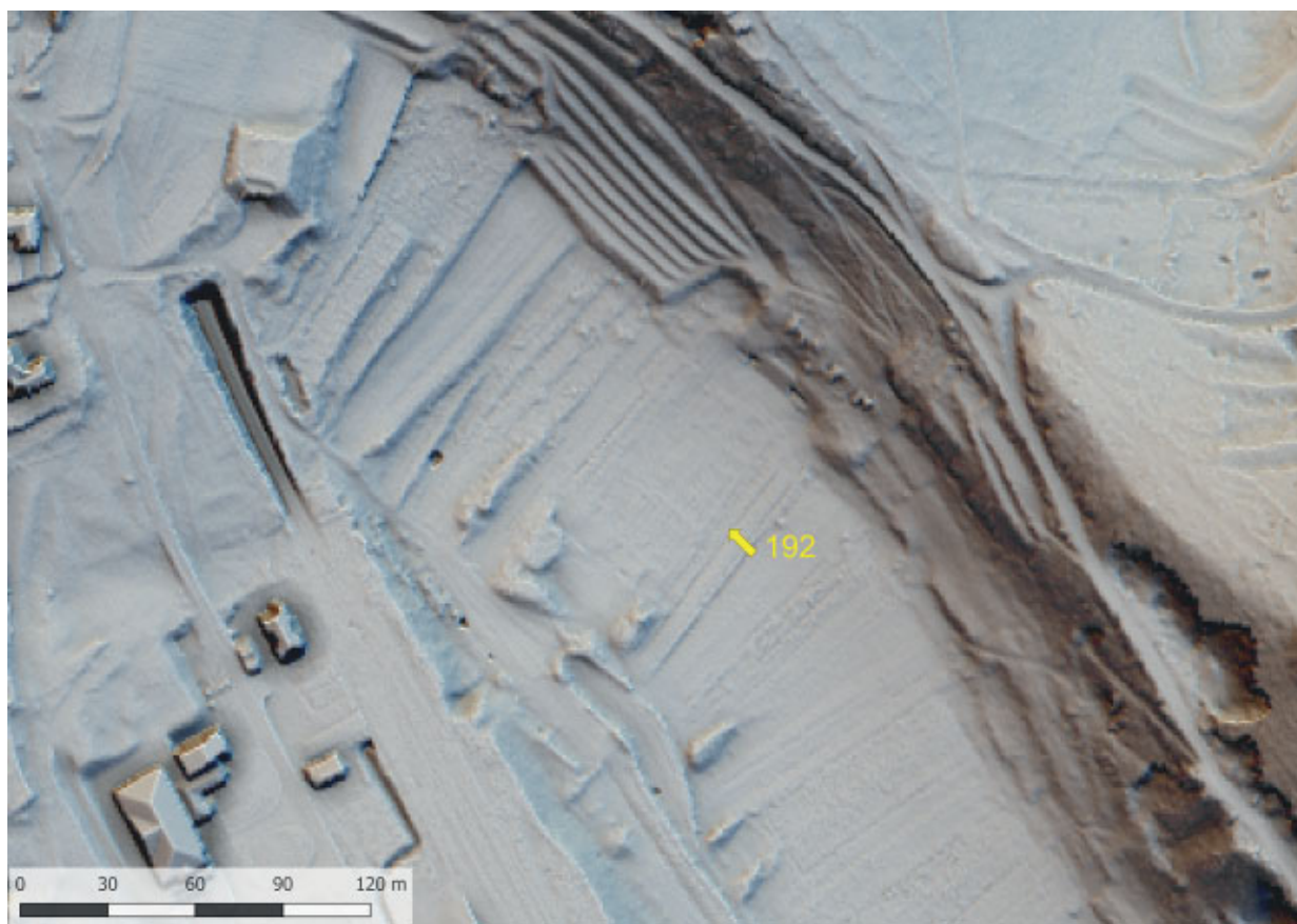
Slika 143 Lidarski posnetek: vojaško pokopališče v Štanjelu (kat. št. 192) (izvedba M. Mori).
