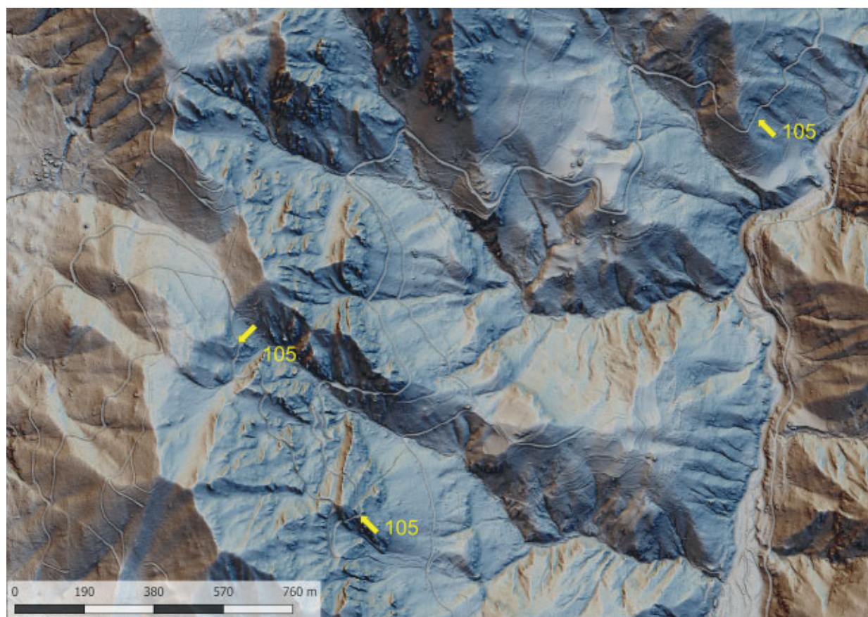
Slika 81 Lidarski posnetek: cesta Dolenja Trebuša–Čepovan (kat. št. 105) (izvedba M. Mori).
