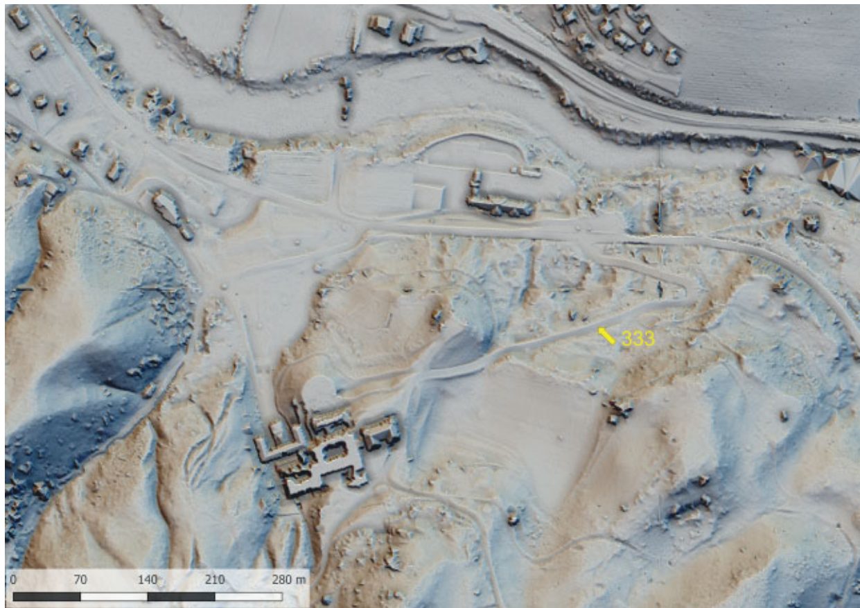
Slika 174 Lidarski posnetek; Ruska steza pod Sofijinim dvorcem v Rimskih toplicah (kat. št. 333) (izvedba M. Mori).
