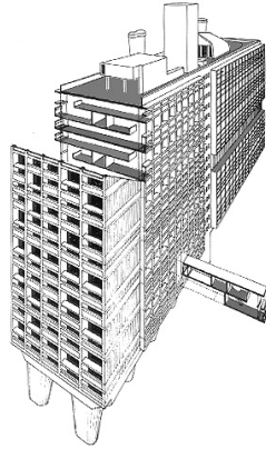
Slika 4: Notranja razporeditev prostorov v bivalni enoti, 3 izdelani na osnovi Le Corbusierjevih študij.
