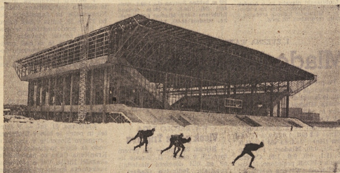
Pokriti ledeni stadion v Tivoliju (Innsbruck), ki je že skoraj povsem zgrajen, bo največje umetno drsalnišče na svetu s površino ledene ploskve okoli 10.800 kvadratnih metrov. V dvorani bo 2000 sedežev in 800 stojišč za gledalce. Pred pokritim ledenim stadionom je steza za hitrostno drsanje, kjer vidimo pri treningu nekaj tekmovalcev. (Posnetki so iz zadnji dni letošnje zime.)
