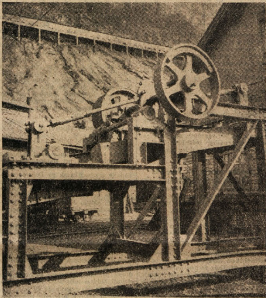
Nihajoče sito za separacijo rudnika Trbovlje-Hrastnik
