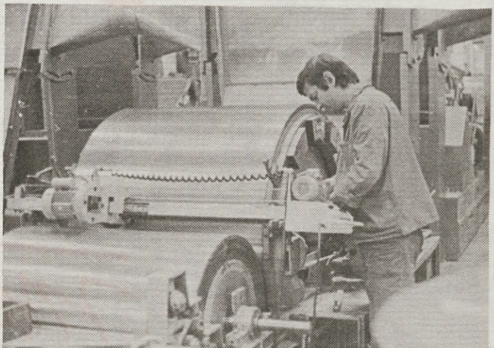
Brusilni stroj od firme Wolters, s katerim natančneje brusimo vse vrste bobnov in gitar pri mikalnikih.
