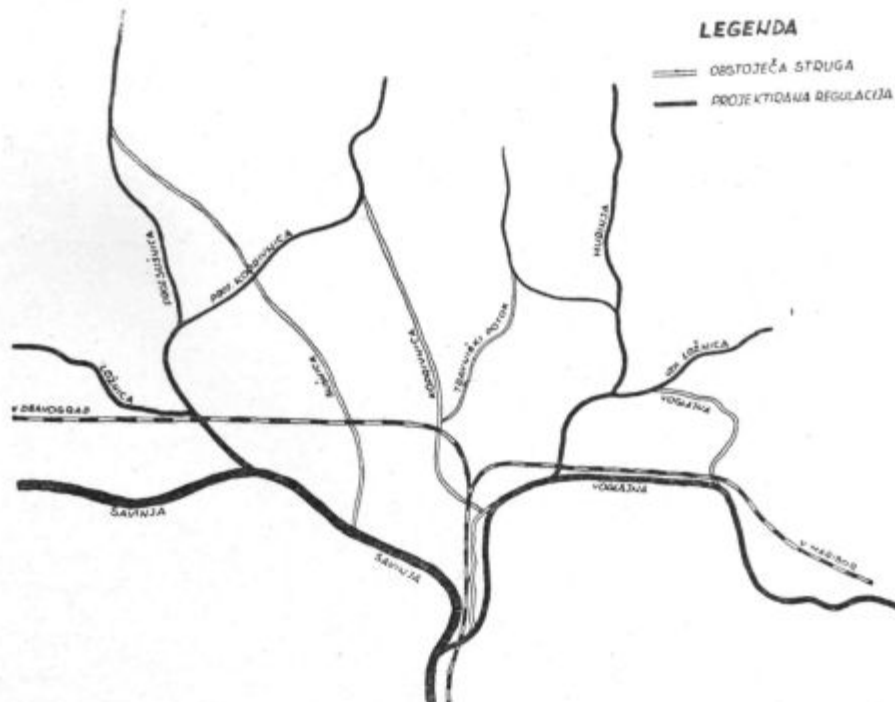
Shema projektiranih regulacij vodnih tokov v celjski kotlini.
