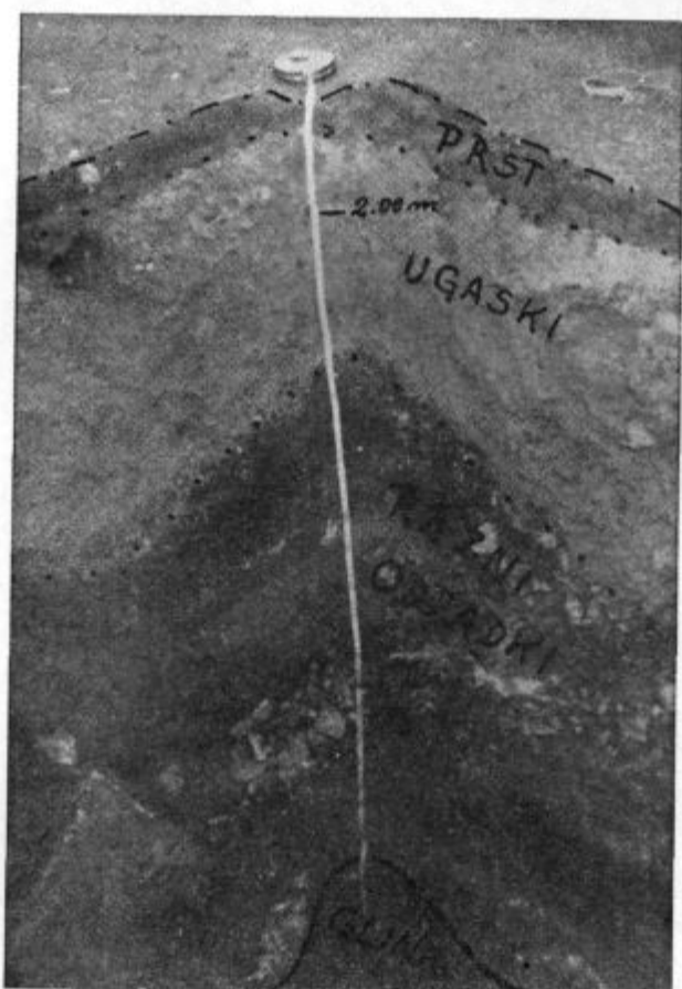
Tipičen profil nasutih tal na severnem robu Celja (sonda v Mestnem mlinu).
