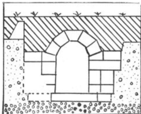
Sl. 3. Prerez severnega kanala v južnih vratih.
