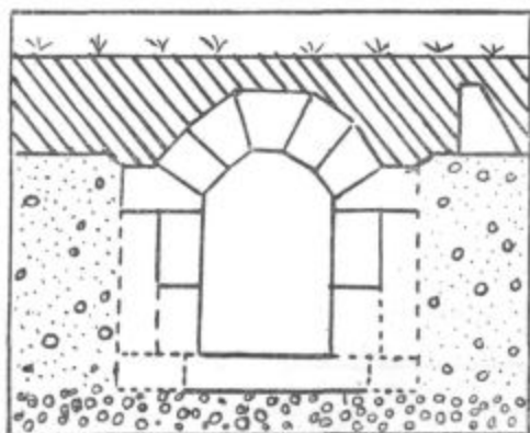
Sl. 2. Prerez južnega kanala v južni vratih.
