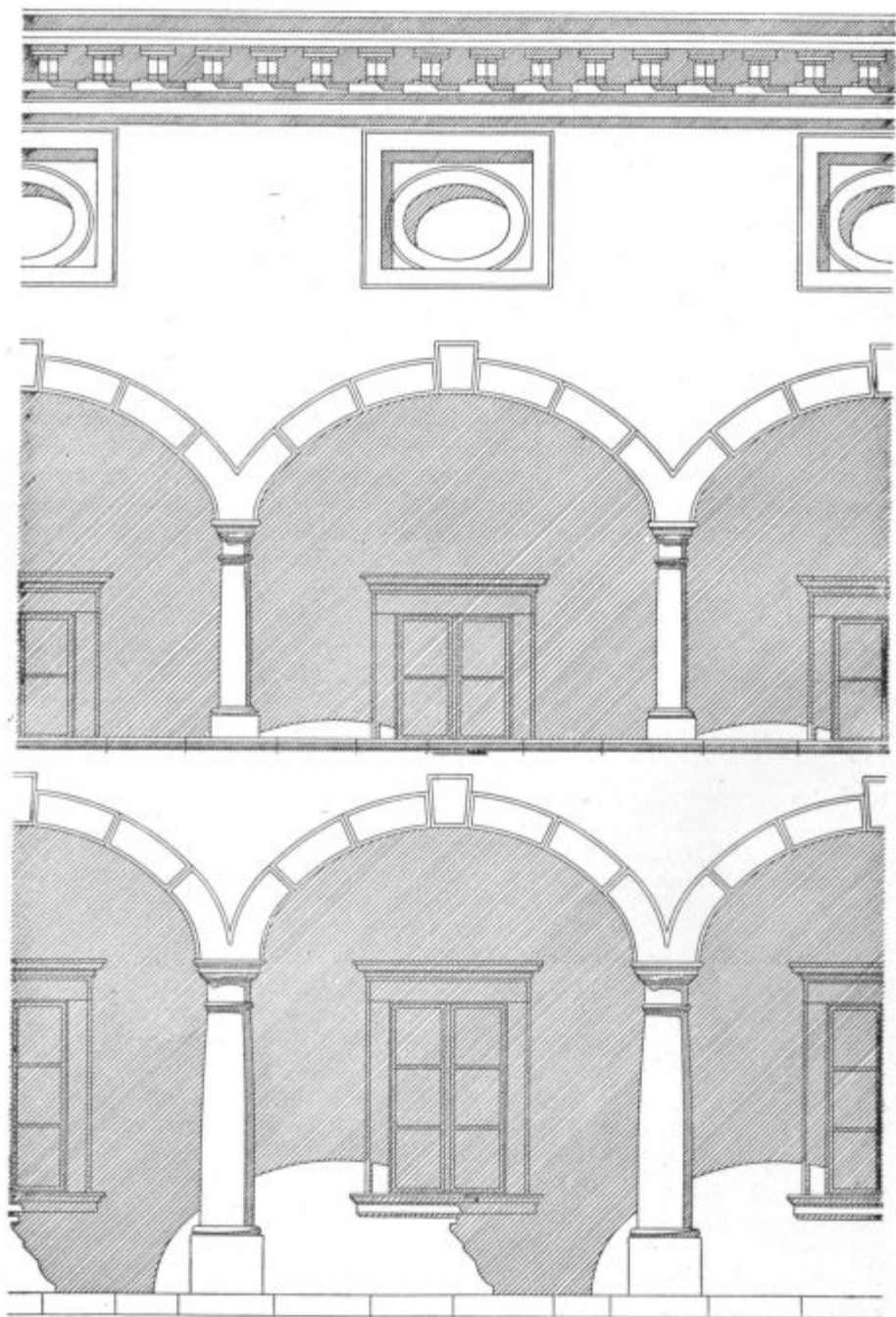
Inž. arh. Marijan Mušič: Detajl restavrirane fasade na severni strani stare grofije.
