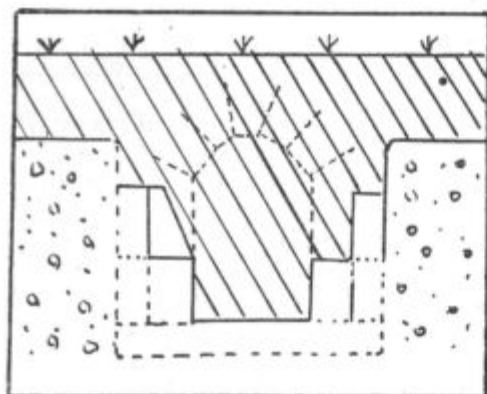
Sl. 4. Prerez kanala v severnih vratih.
