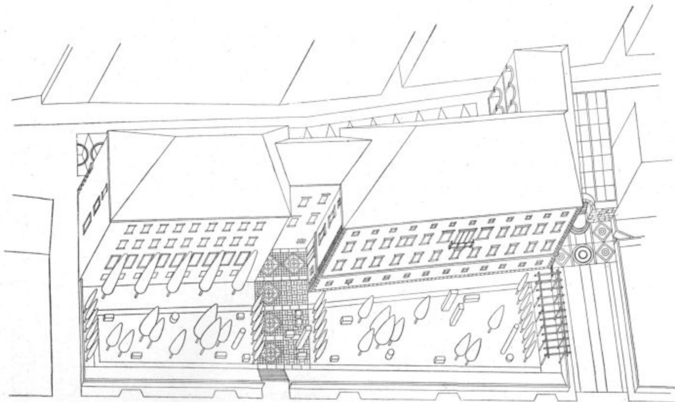
Inž. arh. Marijan Mušič: Aksonometrija obeh poslopij grofije in muzejskega parka ob južni fasadi.
