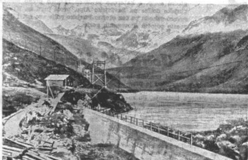
V Avstriji so pravkar dovršili ogromno električno centralo, ki bo oskrbovala z električnim tokom tudi Nemčijo do Porenja. Centrala leži pri ledniku Silvretta in zbira odtoke iz njega v umetnem jezeru, ki je v njem prostora za 5.4 milijonov kubičnih metrov vode. S tem dobi naprava 700 m padca, ki daje zopet električno silo novi centrali Parthenen na Predariskem.
