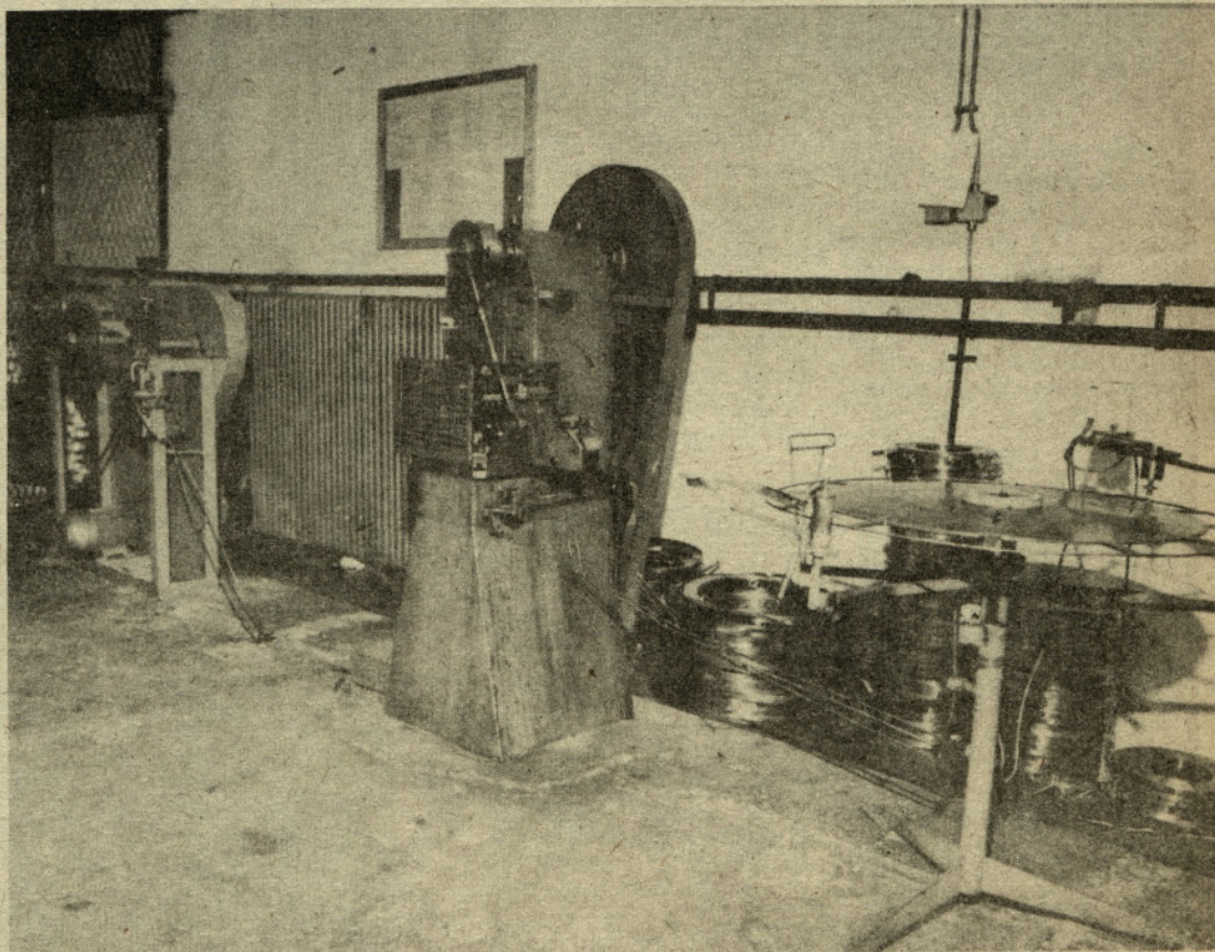
Avtomat, izdelan po lastni konstrukciji v delavnici Jožeta Pevca. Na njem teče avtomatska izdelava sponk
