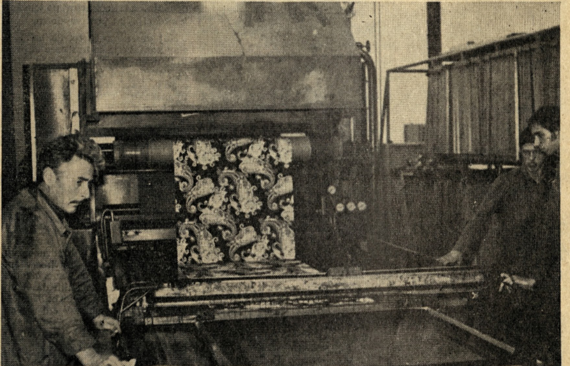
Rotacijski tiskarski stroj STORK v plemenitilnici I
