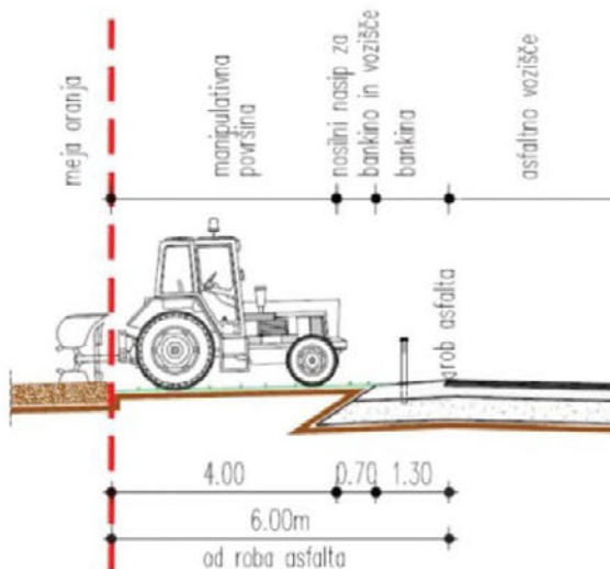
(Vir skice: Oranje pravokotno 90 in vzporedno_Prez. pdf, Cestno podjetje Nova Gorica in Ministrstvo RS za infrastrukturo in prostor)
