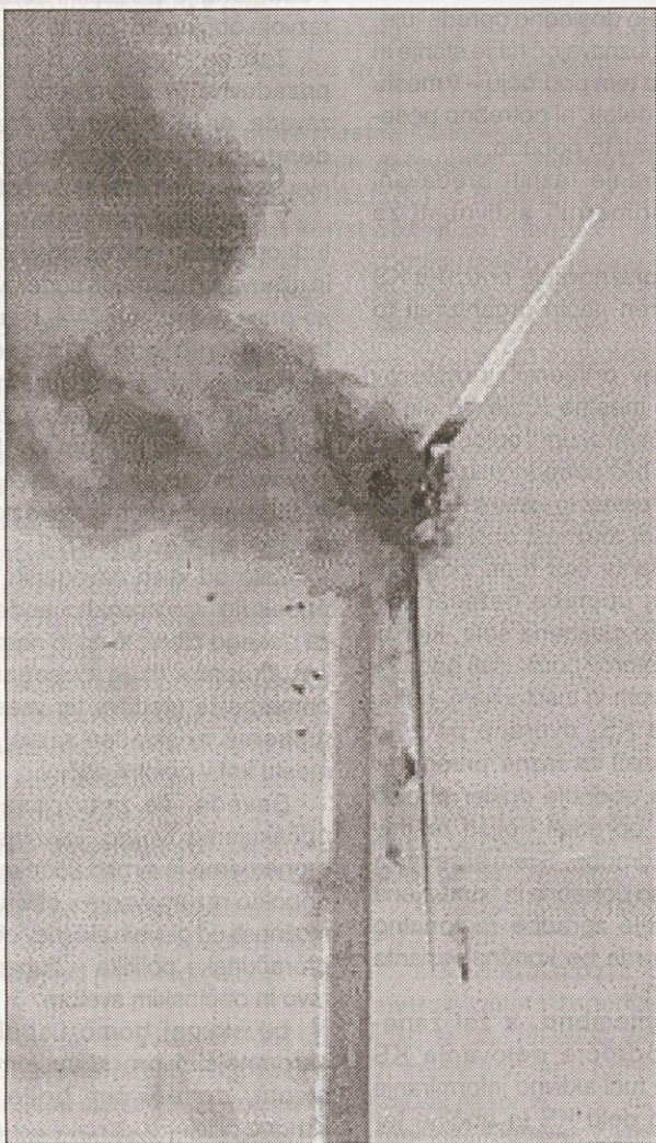
Do požara na turbini lahko pride zaradi okvare na generatorju. Gorljivih materialov je očitno dovolj.
