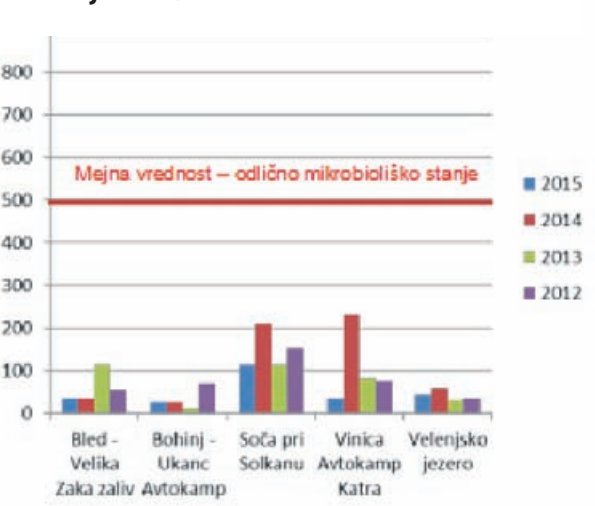
Povprečno število E.Coli bakterij v Velenjskem jezeru in v nekaterih naravnih kopalniščih v obdobju 2012/15
