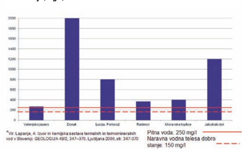
Primerjava povprečne vsebnosti sulfata na površini Velenjskega jezera (2012/15) z nekaterimi vrelni mineralne vode v Sloveniji (mg/l)*
