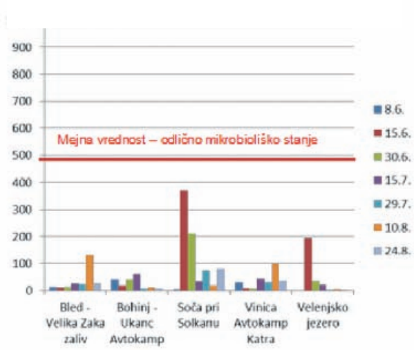
Število E.Coli bakterij v Velenjskem jezeru in v nekaterih naravnih kopalniščih po datumih v letu 2015
