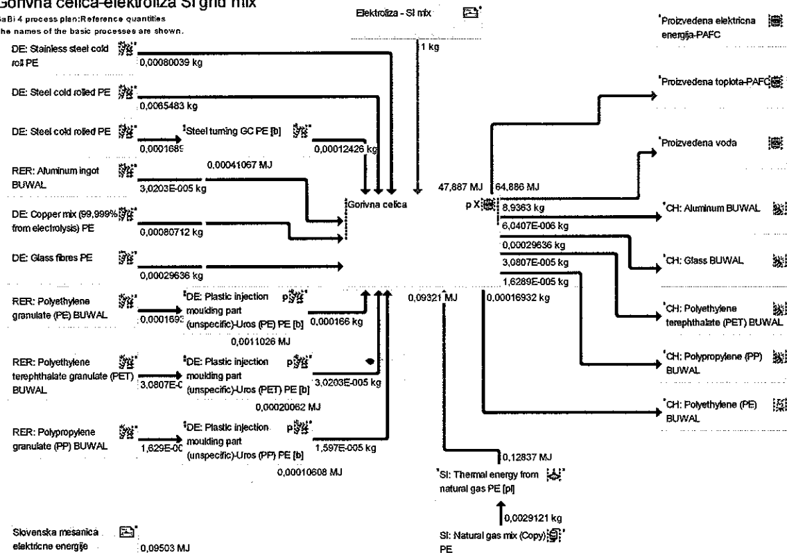
Slika 3.15: Shema obravnavane gorivne celice v GaBi 4
