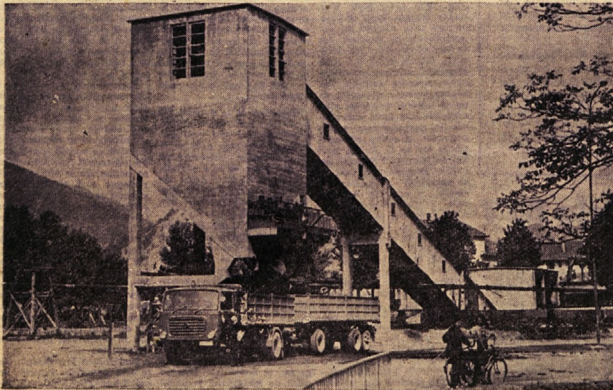
Nova nakladalna postaja (bunker) za premog na obratu Kisovec. S prevozom premoga s tovornjaki s prikolicami so se stroški prevoza premoga znatno zmanjšali.
