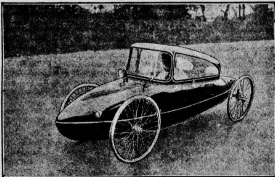
Avtomobil brez motorja. Goni ga kolesar sam. Pritlikavček je zelo udoben in ne stane dosti več kakor navadno kolo. Voditi ga more vsak otrok.
